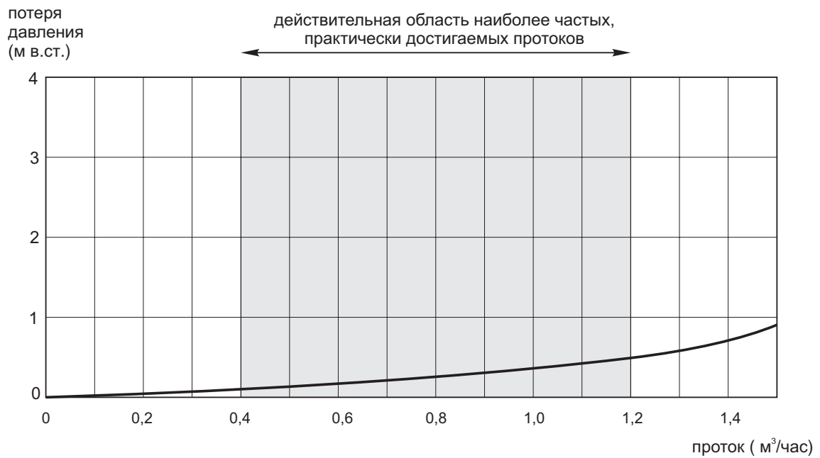
Рис.3 Потери давления бойлера PROTHERM В 100
