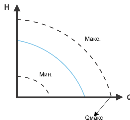
Рис. 49 Q_{\max}
