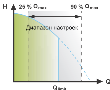
Рис. 45 FLOW LIMIT
