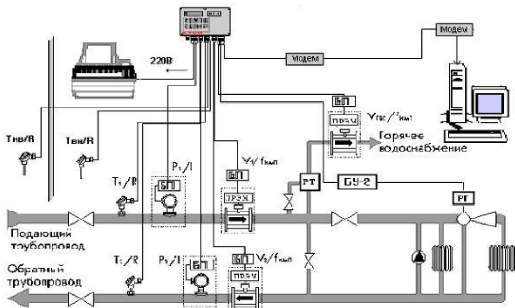
Рис. Функциональная схема системы учета и регулирования теплопотребления
