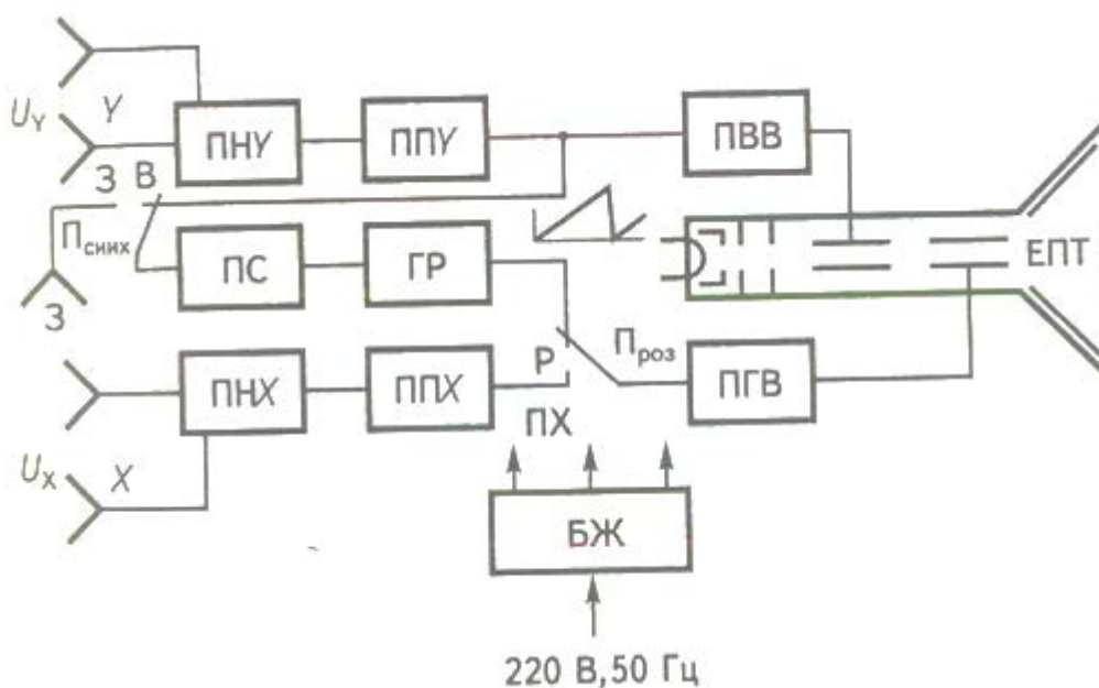
Рисунок 5.5. Структурно-функціональна схема електронно-променевого осцилографа
