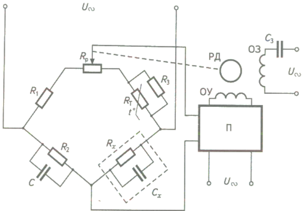
Рисунок 5. Схема автоматичного контактного кондуктометра
