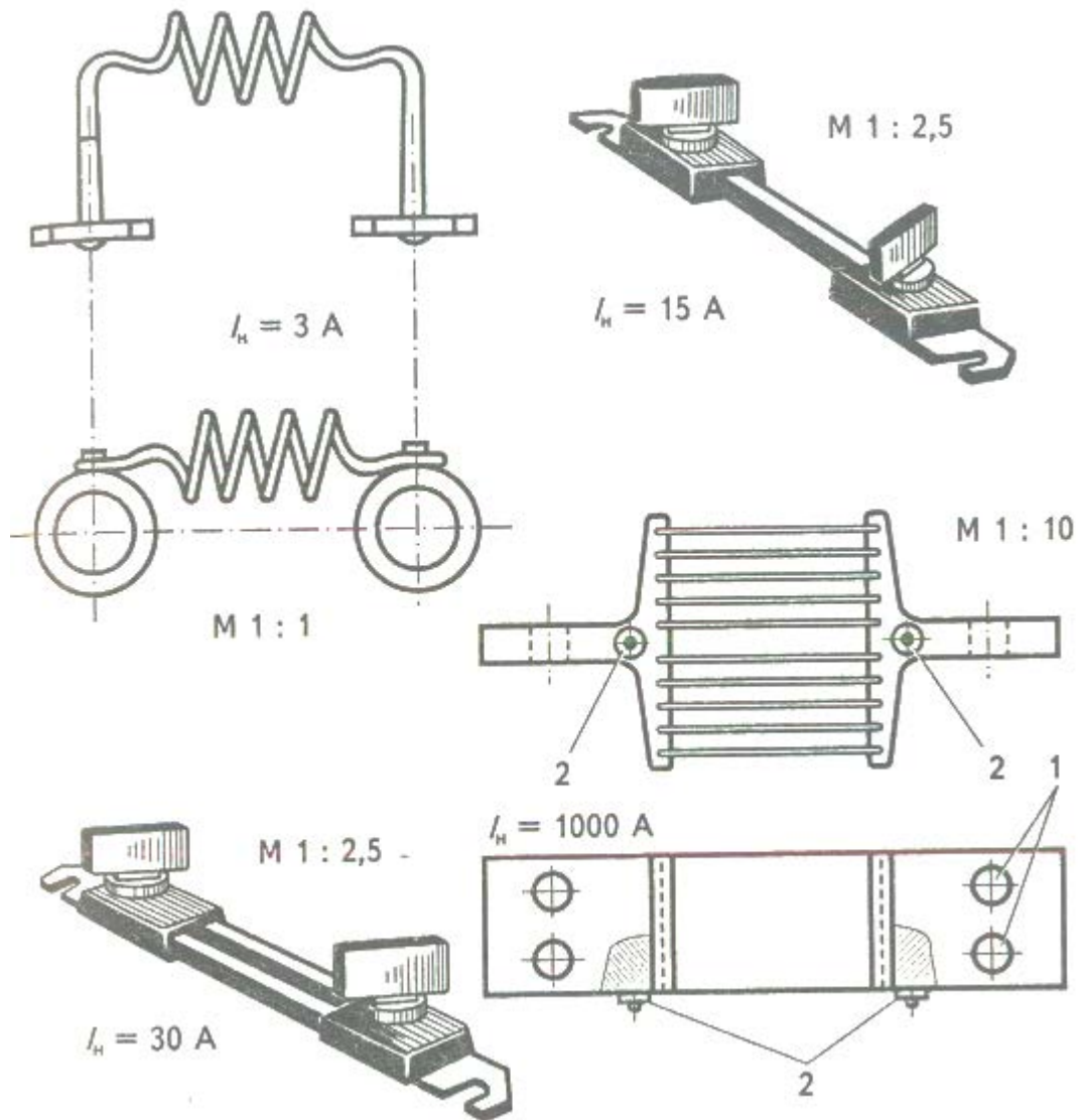
Рисунок 1. Електричні шунти
