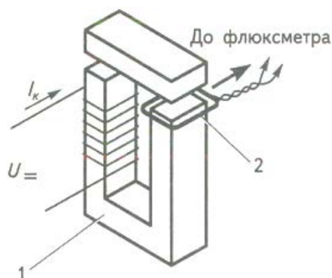
Рисунок 2. Вимірювання величини магнітного потоку електромагніту флюксометром
