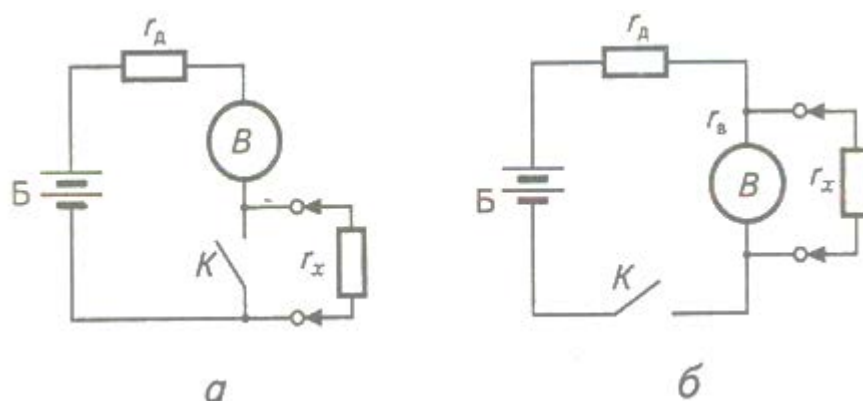
Рисунок 1. Схеми опорів з магнітоелектричними вимірювальними механізмами, що мають регульовані магнітні шунти: a – схема для вимірювання великих опорів; б – схема для вимірювання малих опорів
