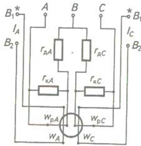
Рисунок 6. Схема переносного трифазного електродинамічного ватметра
