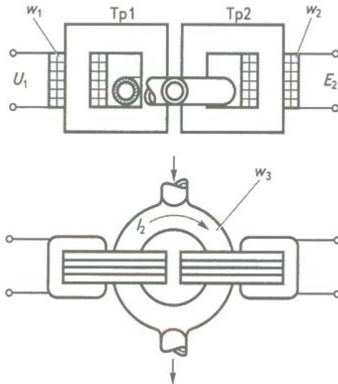
Рисунок 6. Чутливий елемент безконтактного концентратоміра
