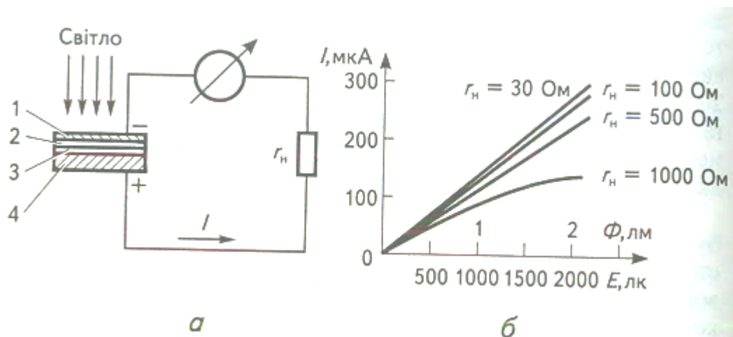
Рисунок 12. Вентильний фотоелемент: а – будова фотоелемента; б – світлова характеристика
