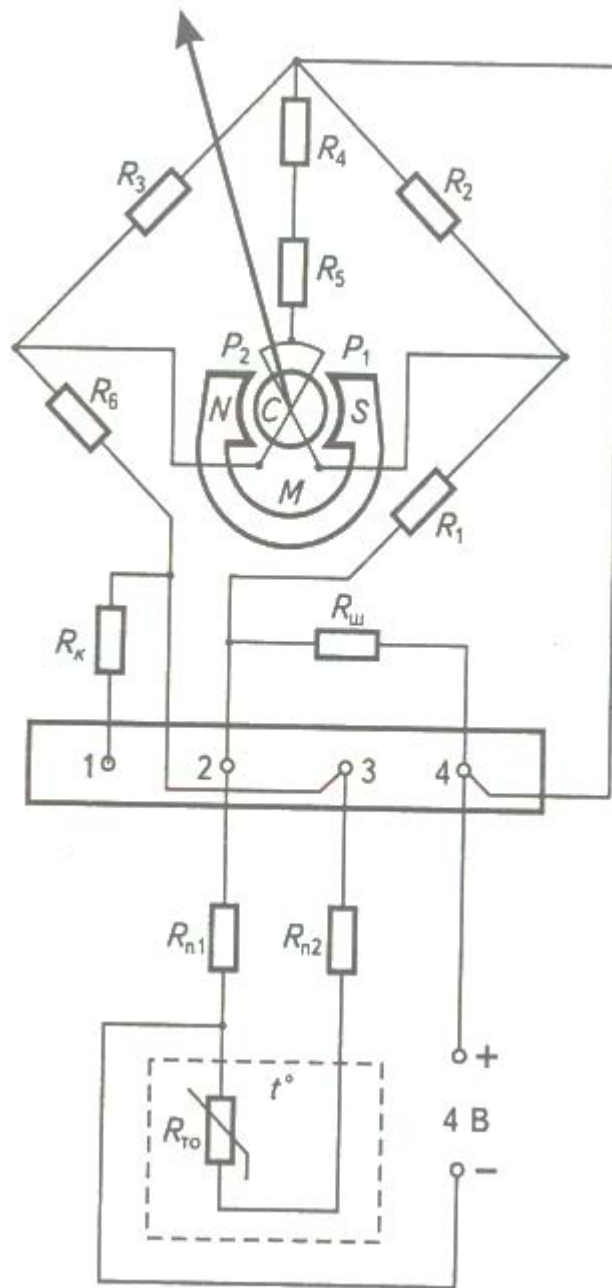
Рисунок 1. Принципова електрична схема логометра з терморетворювачем опору
