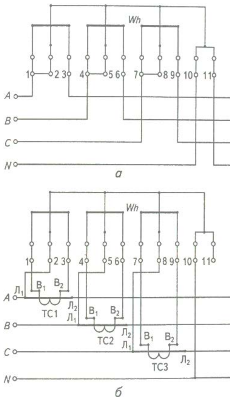
Рисунок 5. Схеми вмикання трифазних трьохелементних лічильників: a – пряме для вимірювання в колі з несиметричним навантаженням; б – за допомогою трансформаторів струму
