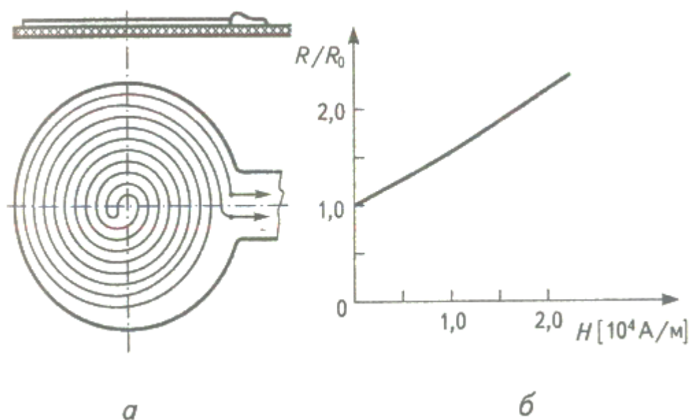
Рисунок 3. Вісмутова спіраль для визначення величини напруженості магнітного поля: a – конструкція спіралі; б – залежність величини опору спіралі від напруженості магнітного поля
