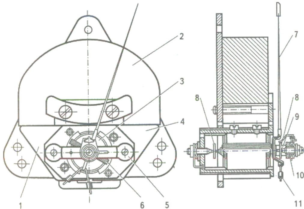
Рисунок 1. Вимірювальний механізм магнітоелектричної системи
