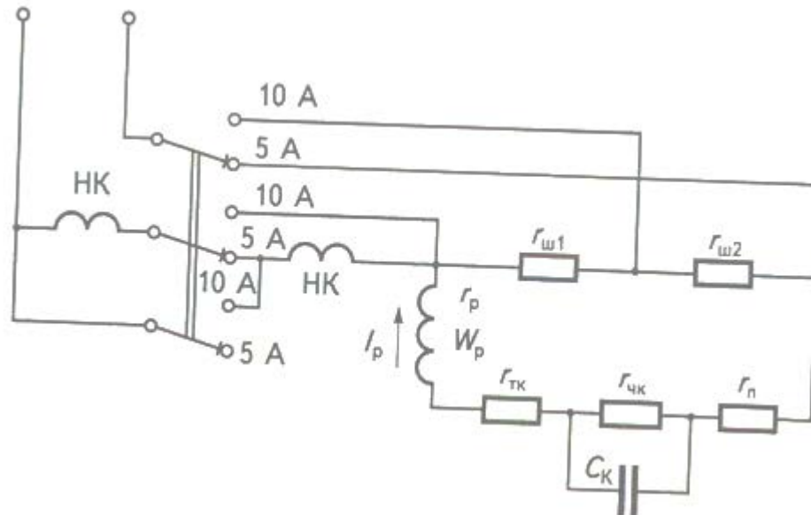
Рисунок 3. Принципові схеми електродинамічного амперметра
