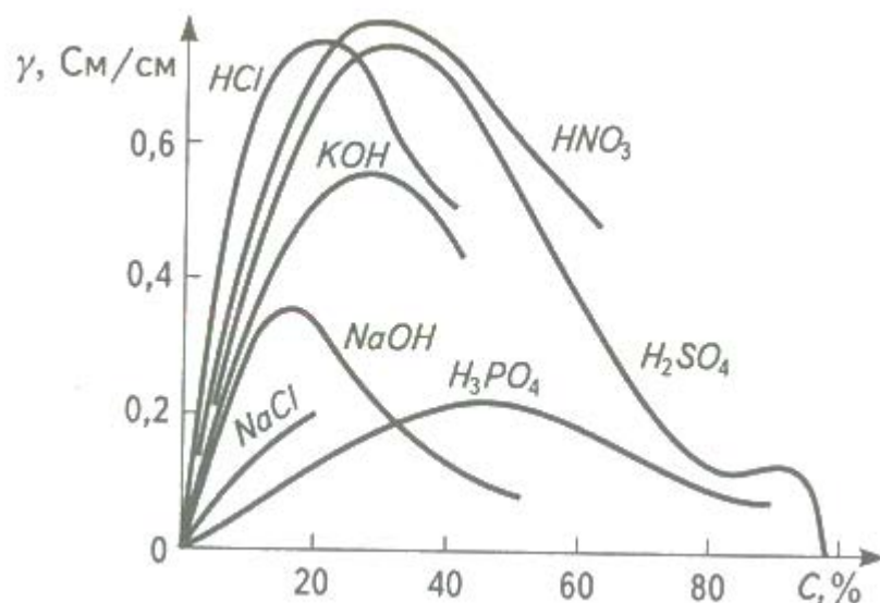
Рисунок 4. Залежності питомої електропровідності розчинів від концентрації (температура 20 °С)
