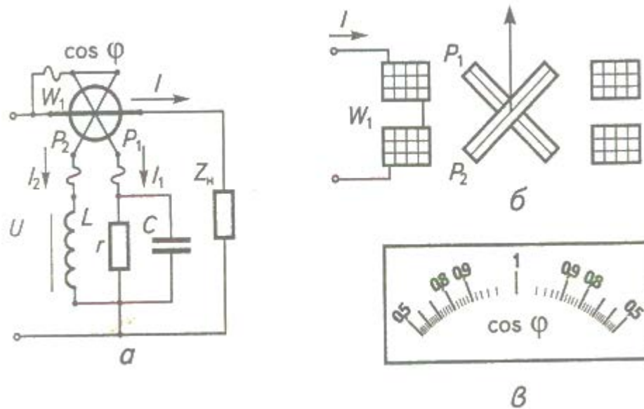
Рисунок 1. Однофазний електродинамічний фазометр: a – принципова схема; б – будова вимірювального механізму; в – шкала
