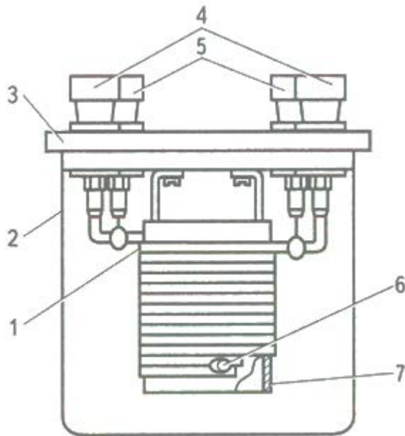
Рисунок 3.2. Зразкова котушка опору
