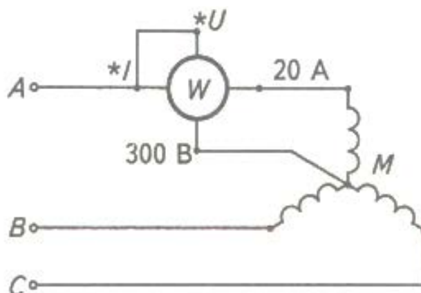
Рисунок 7. Схема вимірювання потужності, споживаної трифазним двигуном, однофазним ватметром
