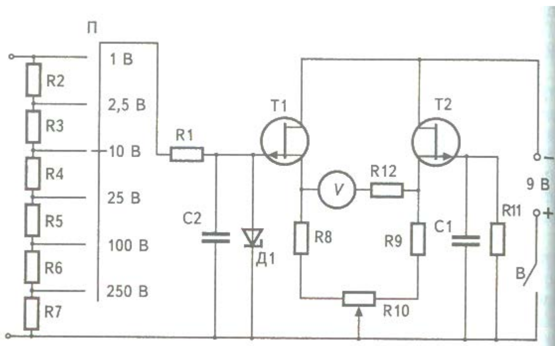
Рисунок 5.2. Схема електронного вольтметра на польових транзисторах
