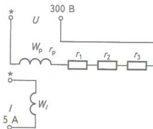
Рисунок 1. Схема стаціонарного ватметра
