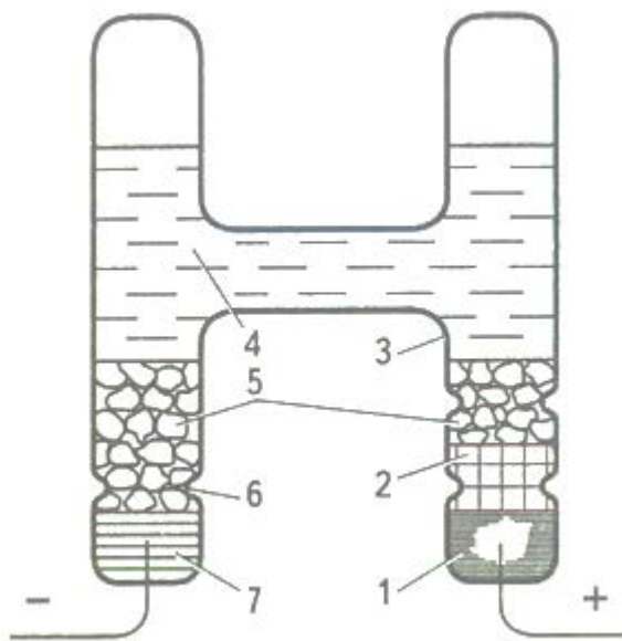
Рисунок 3.1. Будова насиченого нормального елемента
