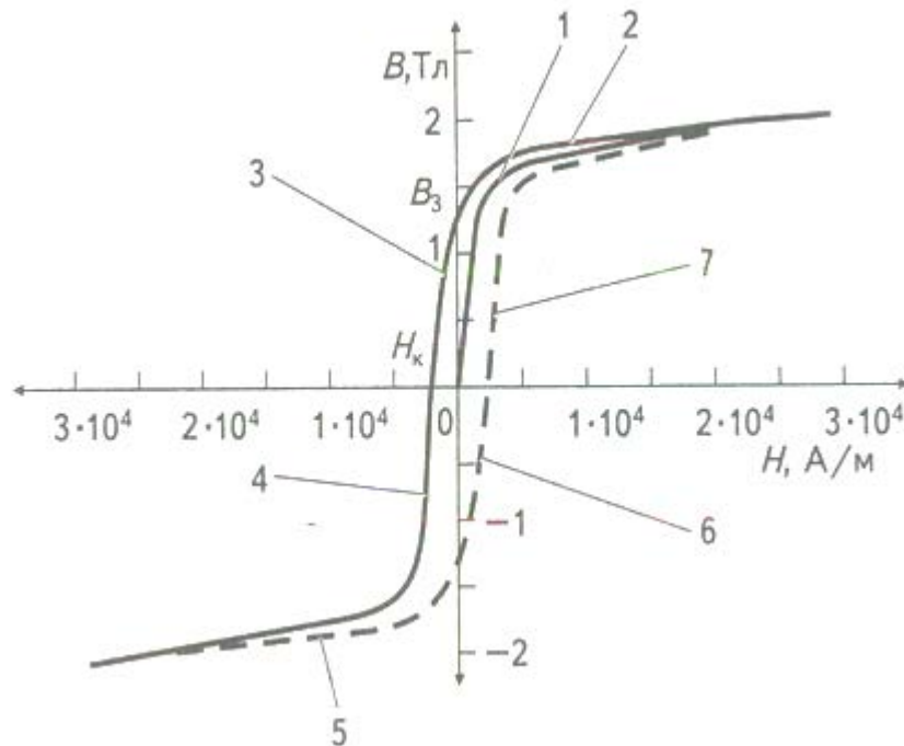
Рисунок 6. Характеристики намагнічування ферромагнітного матеріалу і петля гістерезису
