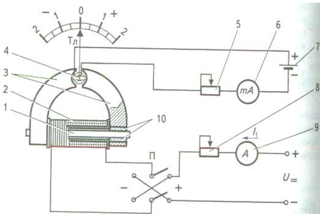
Рисунок 5 Пермеаметр
