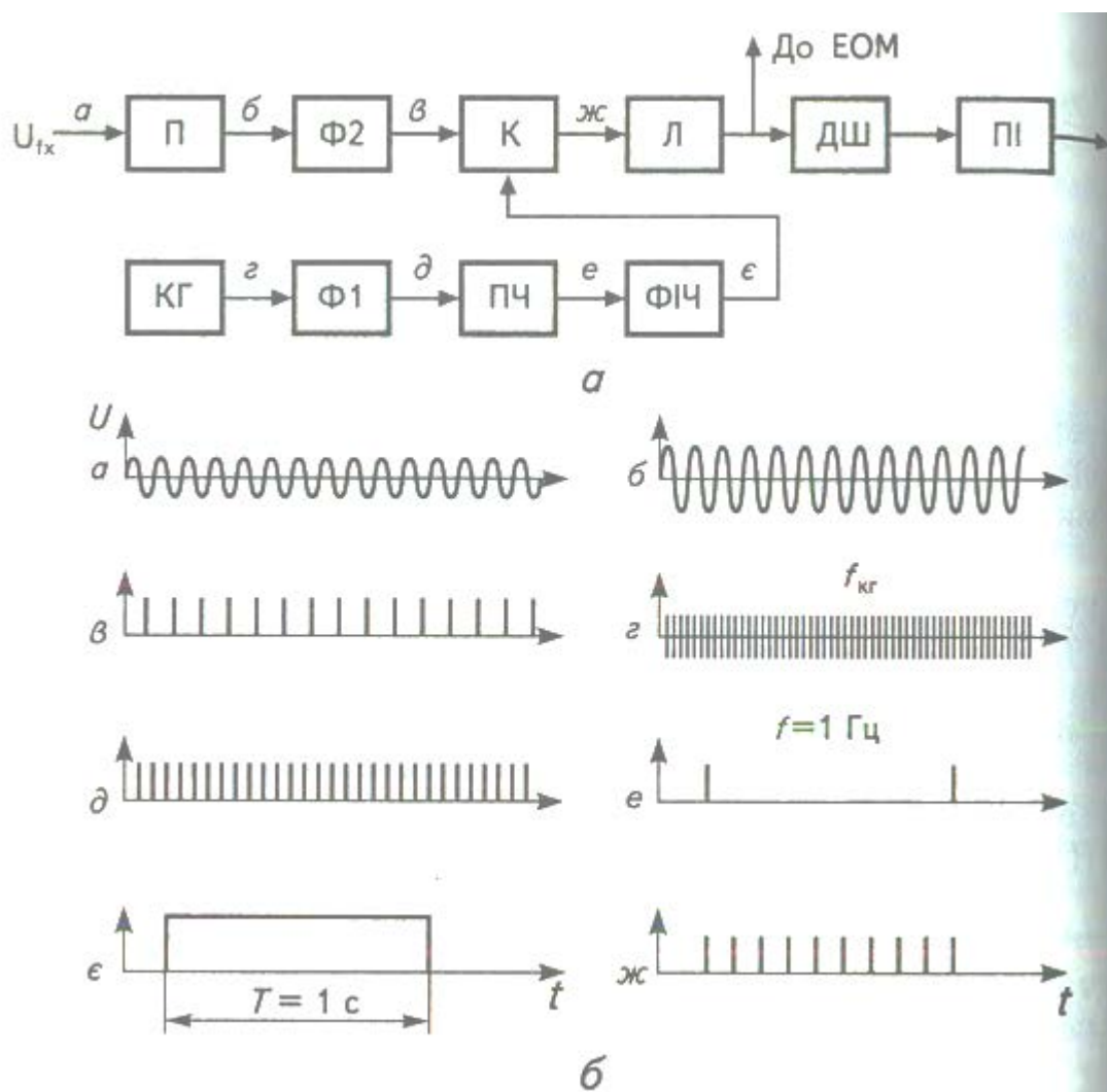
Рисунок 4. Структурно-функціональна схема цифрового частотоміра: а – схема; б – епюри напруг
