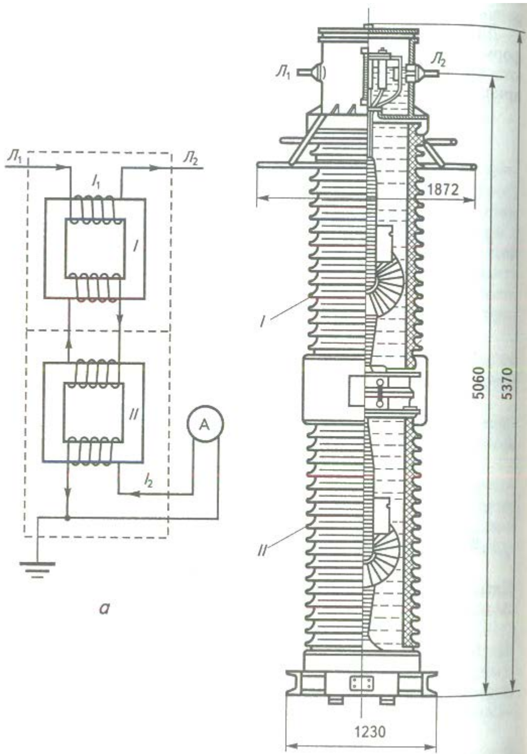
Рисунок 6. Каскадний трансформатор струму: а – схема; б – будова
