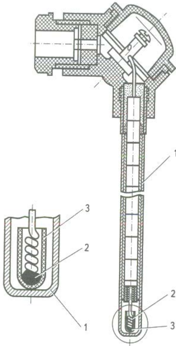
Рисунок 7. Термопара з арматурою
