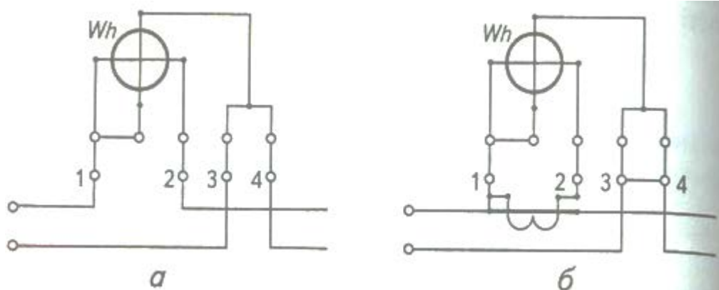
Рисунок 2. Схеми вмикання однофазних лічильників: a – пряме вмикання в мережу; б – вмикання через вимірювальний трансформатор струму
