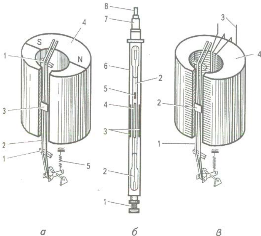
Рисунок 7. Вібратори електромеханічних осцилографів: а – петльовий; б – рамковий; в – потужності
