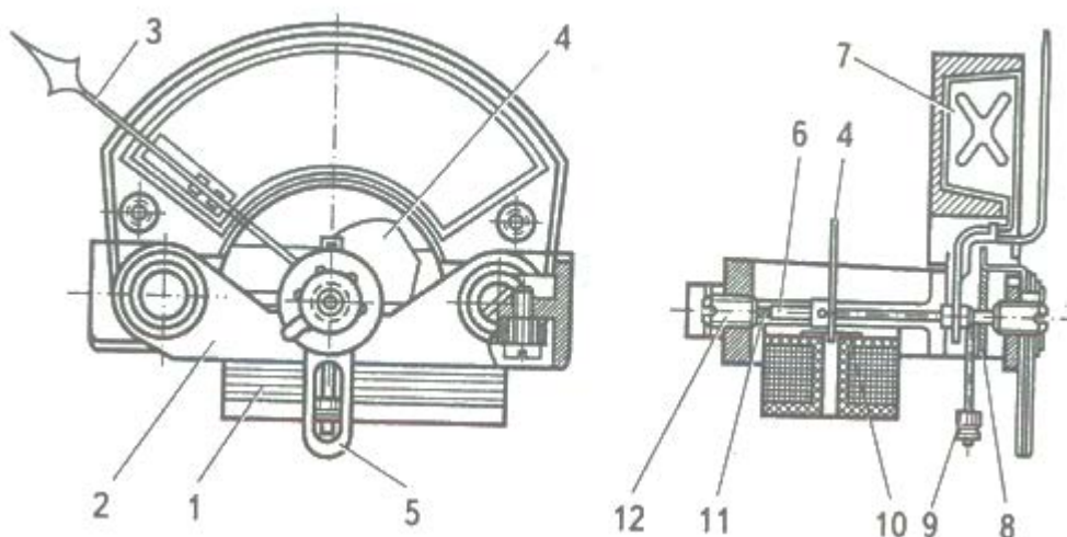
Рисунок 2. Вимірювальний механізм електромагнітної системи
