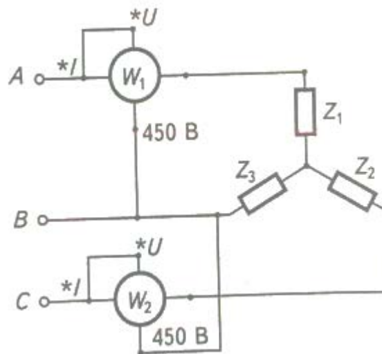
Рисунок 9. Схема вимірювання потужності у трифазному три провідному колі двома однофазними ватметрами
