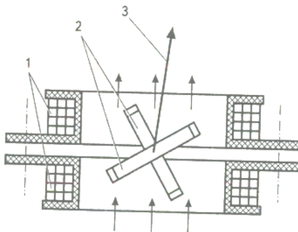
Рисунок 10. Вимірювальний механізм електродинамічного логометра
