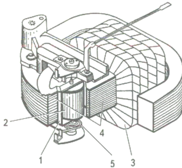
Рисунок 4. Вимірювальний механізм феродинамічної системи
