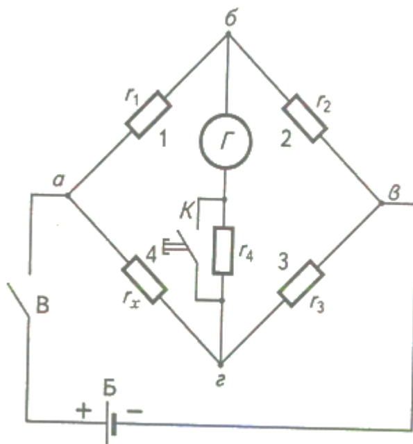
Рисунок 5. Схема мосту для вимірювання опорів
