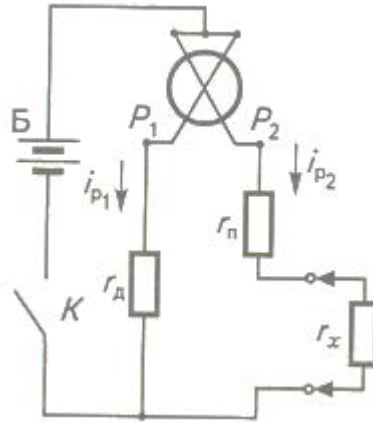
Рисунок 3. Схема омметра, виконана на основі магнітоелектричного логометра
