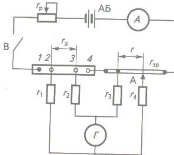
Рисунок 6. Схема вимірювання малих опорів подвійним мостом
