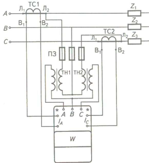
Рисунок 5. Схема вимірювання потужності трифазного кола трифазним ватметром із застосуванням вимірювальних трансформаторів струму і напруги
