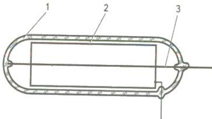
Рисунок 13. Іонізаційний лічильник
