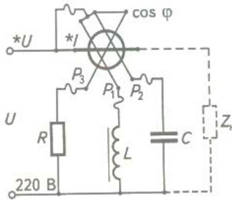
Рисунок 2. Схема однофазного електродинамічного фазометра з компенсацією впливу зміни частоти напруги на показання приладу
