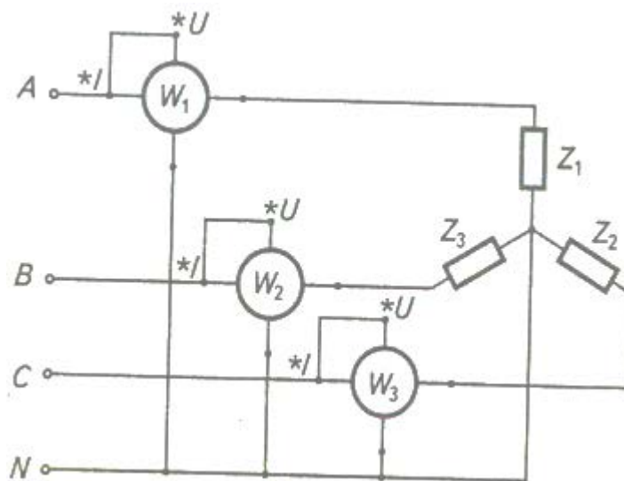
Рисунок 10. Схема вимірювання потужності у трифазному чотири провідному колі трьома однофазними ватметрами
