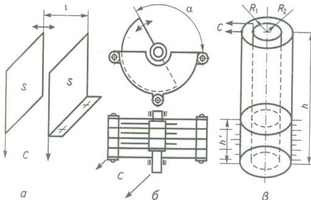
Рисунок 6. Ємнісні перетворювачі
