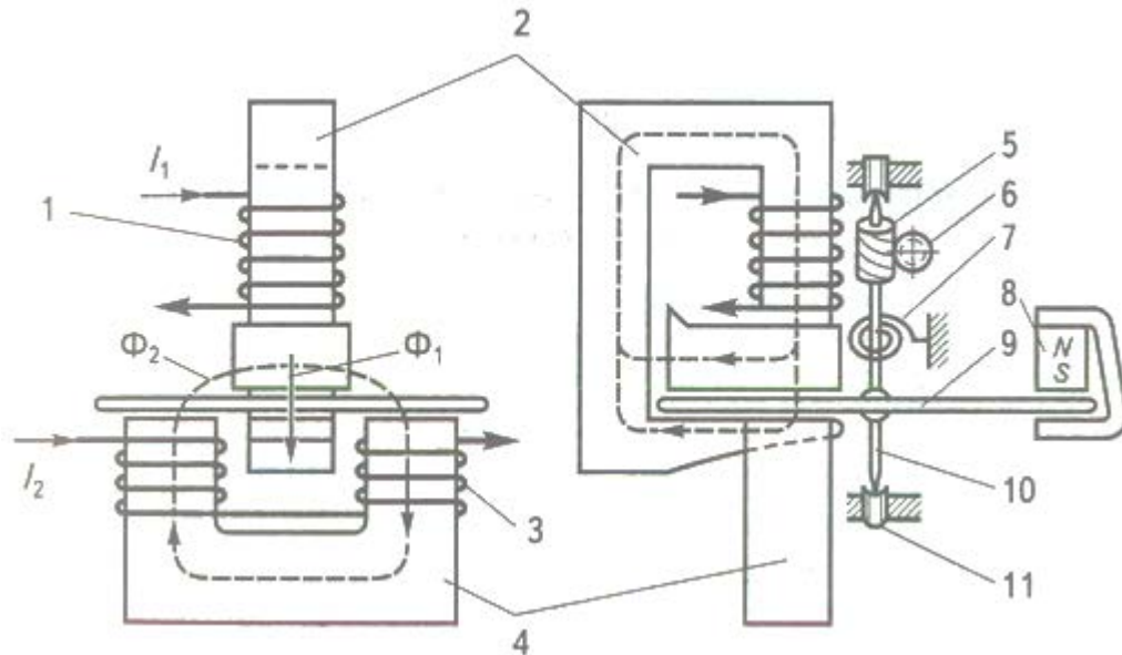
Рисунок 5. Вимірювальний механізм індукційної системи
