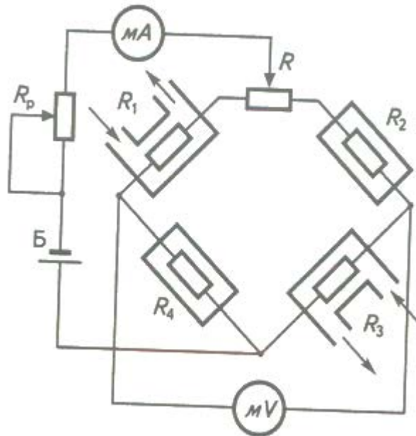
Рисунок 3. Принципова схема термокондуктометричного газоаналізатора
