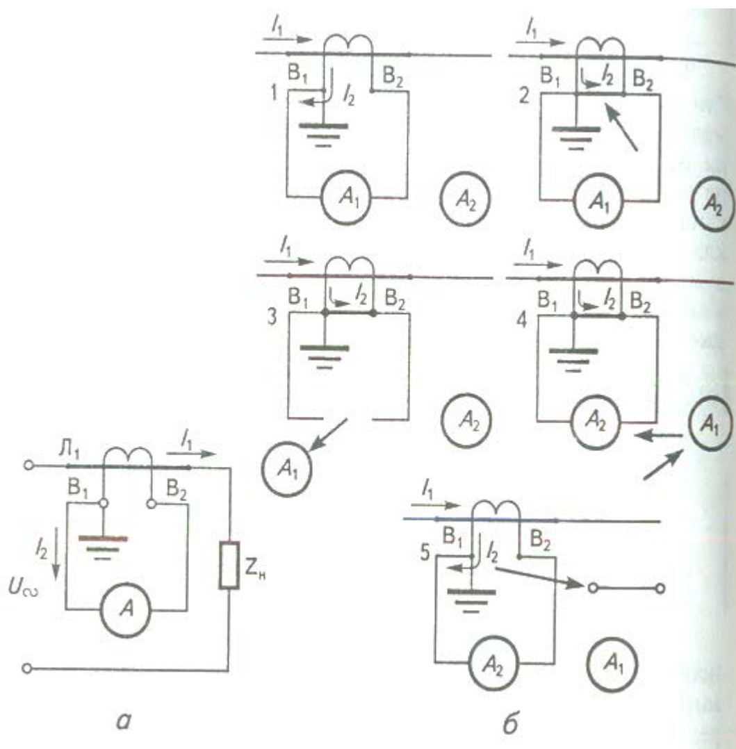
Рисунок 7. Схема вмикання вимірювального трансформатора струму: а – схема вмикання для вимірювань; б – порядок дій при заміні амперметра у вторинному комі трансформатора
