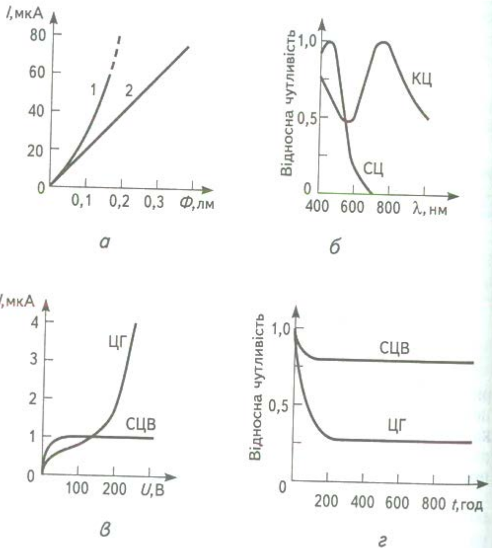
Рисунок 11. Характеристики фотоелементів із зовнішнім фотоелементом: а – світлова; б – спектральна; в – вольт-амперна; г – старіння
