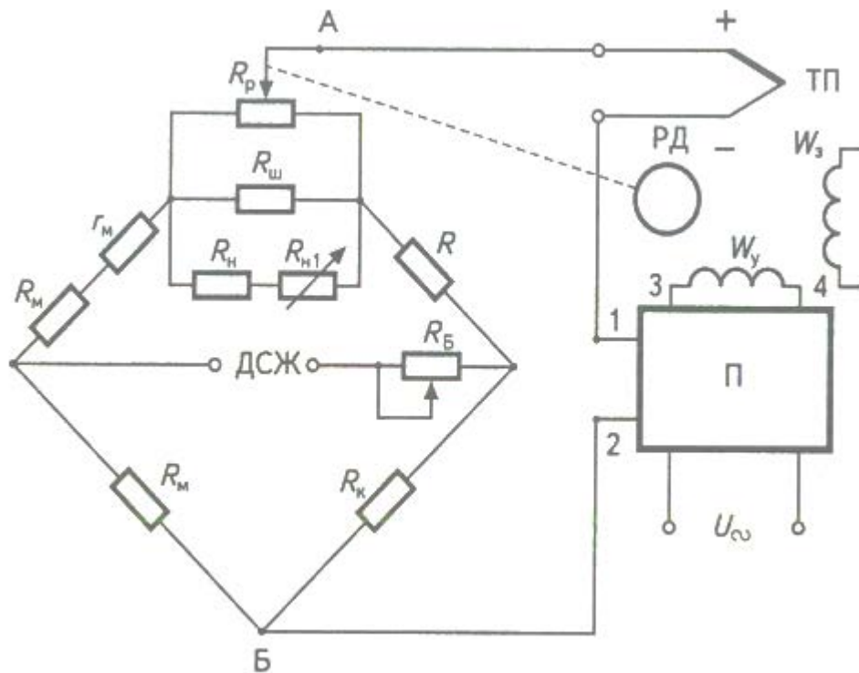
Рисунок 4. Принципова схема для вимірювання ЕРС термопари автоматичним потенціометром
