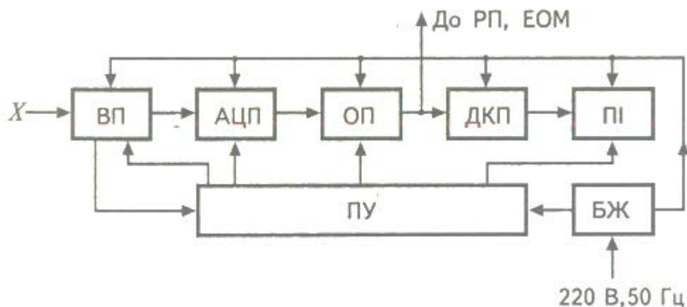
Рисунок 1. Структурна схема цифрового приладу
