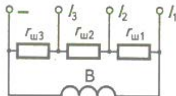
Рисунок 2. Схема магнітоелектричного амперметра
