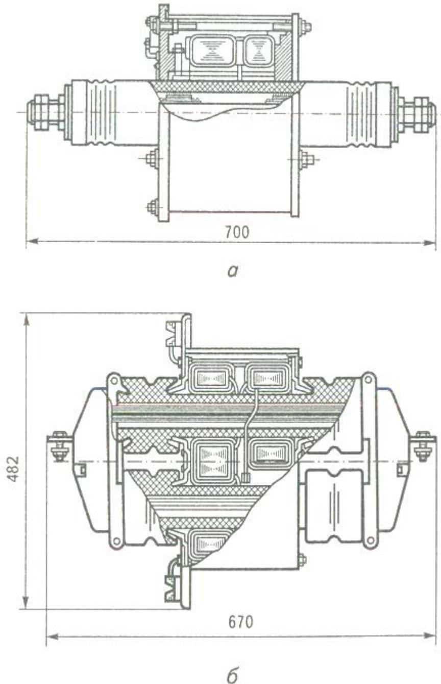
Рисунок 5. Провідні вимірювальні трансформатори струму
