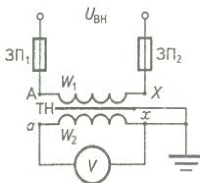
Рисунок 8. Схема ввімкнення вимірювального трансформатора напруги
