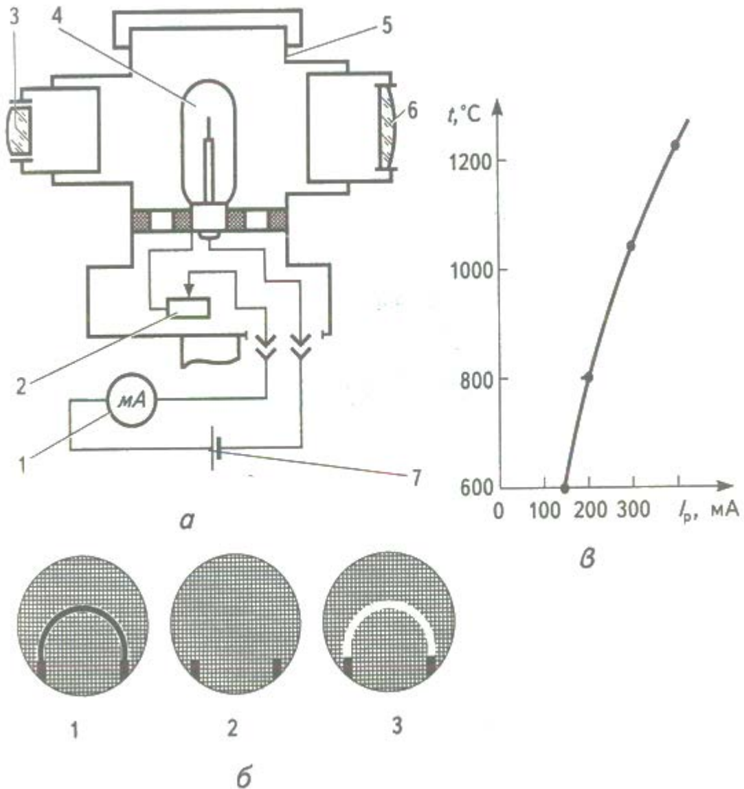
Рисунок 5. Оптичний пірометр: а – будова; б – можливі зображення нитки фотометричної лампи при різних величинах струму в нитці; в – залежність температури нитки від величини струму розжарювання
