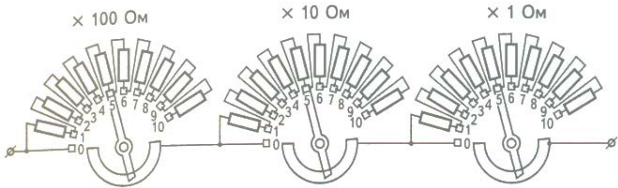
Рисунок 3.4. Будова важільного магазина опорів
