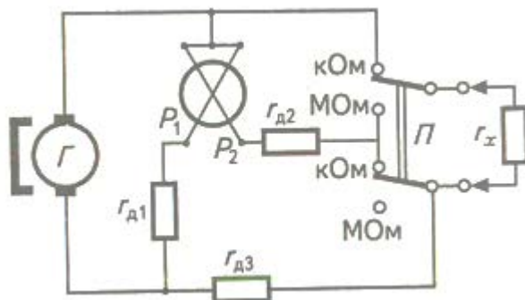
Рисунок 4. Схема мегомметра
