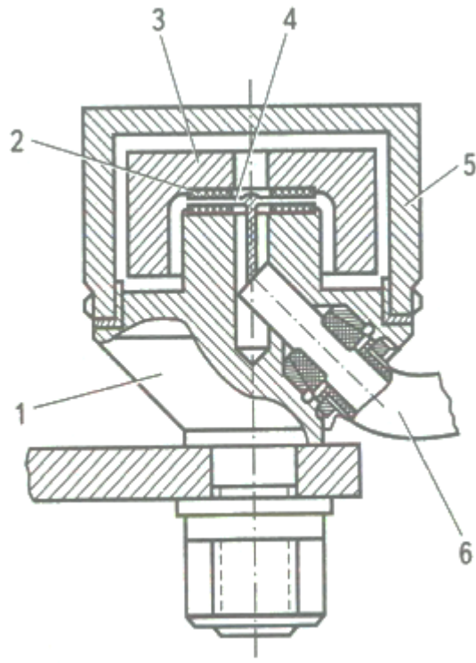
Рисунок 1. П'єзоелектричний акселерометр: 1 – основа; 2 – п'єзокерамічні кільця; 3 – вимірна маса; 4 – контактний диск; 5 – захисний кожух; 6 – екранований кабель
