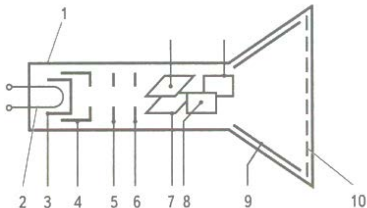
Рисунок 5.4. Будова електронно-променевої трубки з електростатичним відхиленням променя
