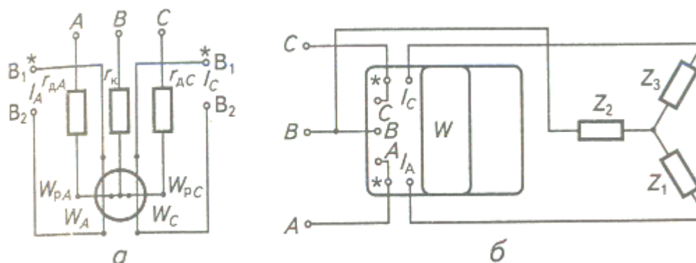
Рисунок 4. Схема стаціонарного трифазного феродинамічного ватметра: а – принципова схема приладу; б – схема вмикання ватметра для вимірювань
