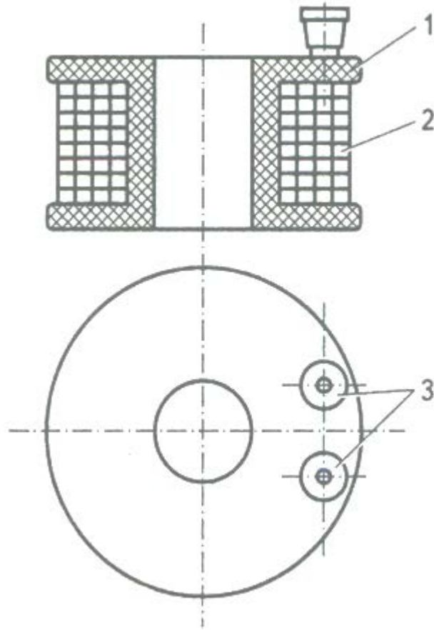
Рисунок 3.5. Котушка індуктивності
