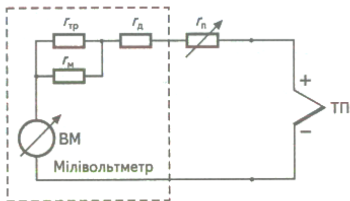
Рисунок 3. Принципова схема з'єднання термопарі з мілівольтметром
