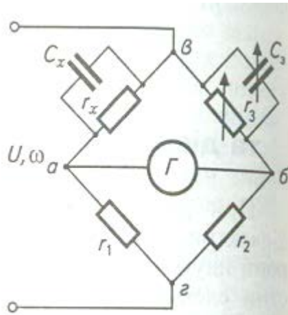
Рисунок 3. Схема моста для вимірювання величин ємностей конденсаторів, що мають значні діелектричні втрати
