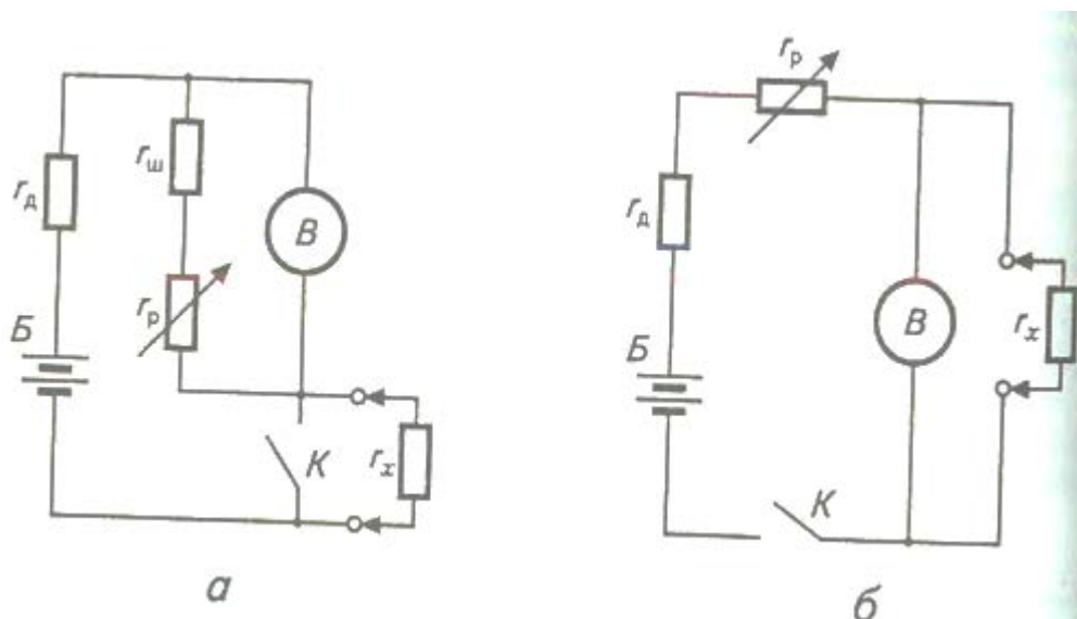
Рисунок 2. Схеми омметрів з регульованими опором: а – схема для вимірювання великих опорів; б – схема для вимірювання малих опорів
