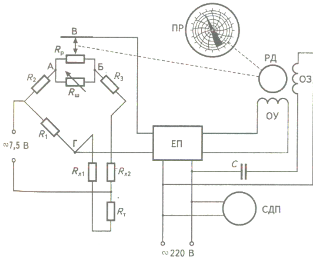
Рисунок 5. Схема автоматичного електронного врівноваженого мосту
