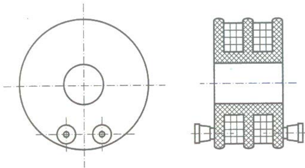
Рисунок 3.6. Котушка взаємоіндуктивності
