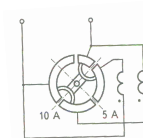
Рисунок 1. Схема двогранчного електромагнітного амперметра
