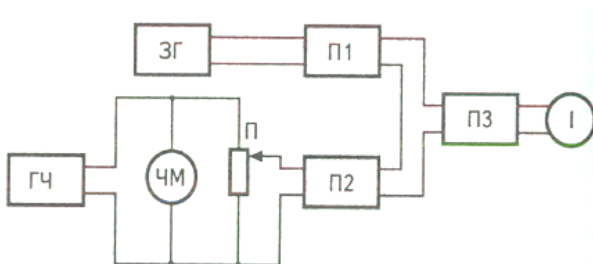
Рисунок 3. Точне вимірювання частоти методом биття
