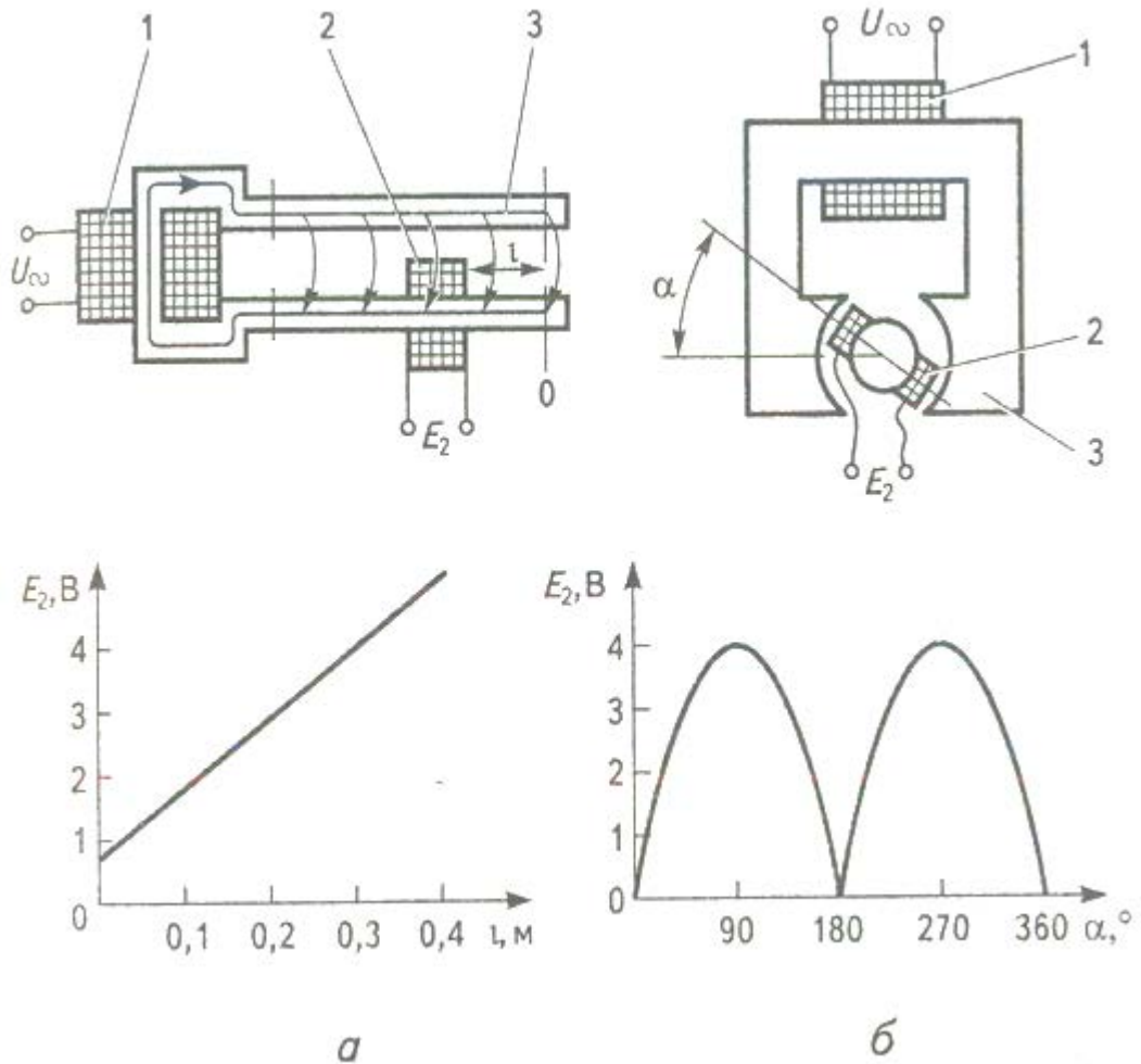
Рисунок 5. Взаємоіндуктивні перетворювачі
