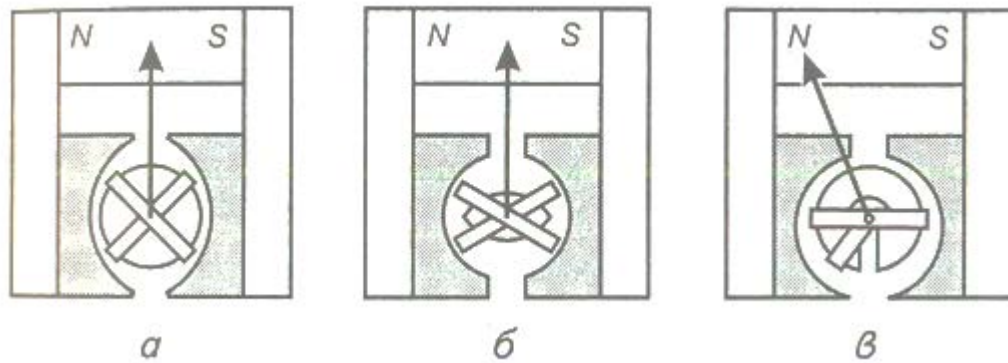
Рисунок 9. Вимірювальні механізми магнітоелектричних логометрів
