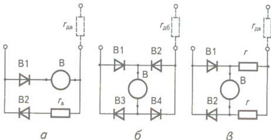
Рисунок 5. Принципові схеми випрамних приладів: а – з однопівперіодним випрямлячем; б, в – з двопівперіодним випрямлячем
