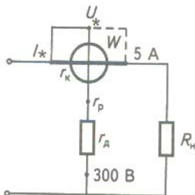
Рисунок 3. Схема вмикання ватметра для вимірювання потужності
