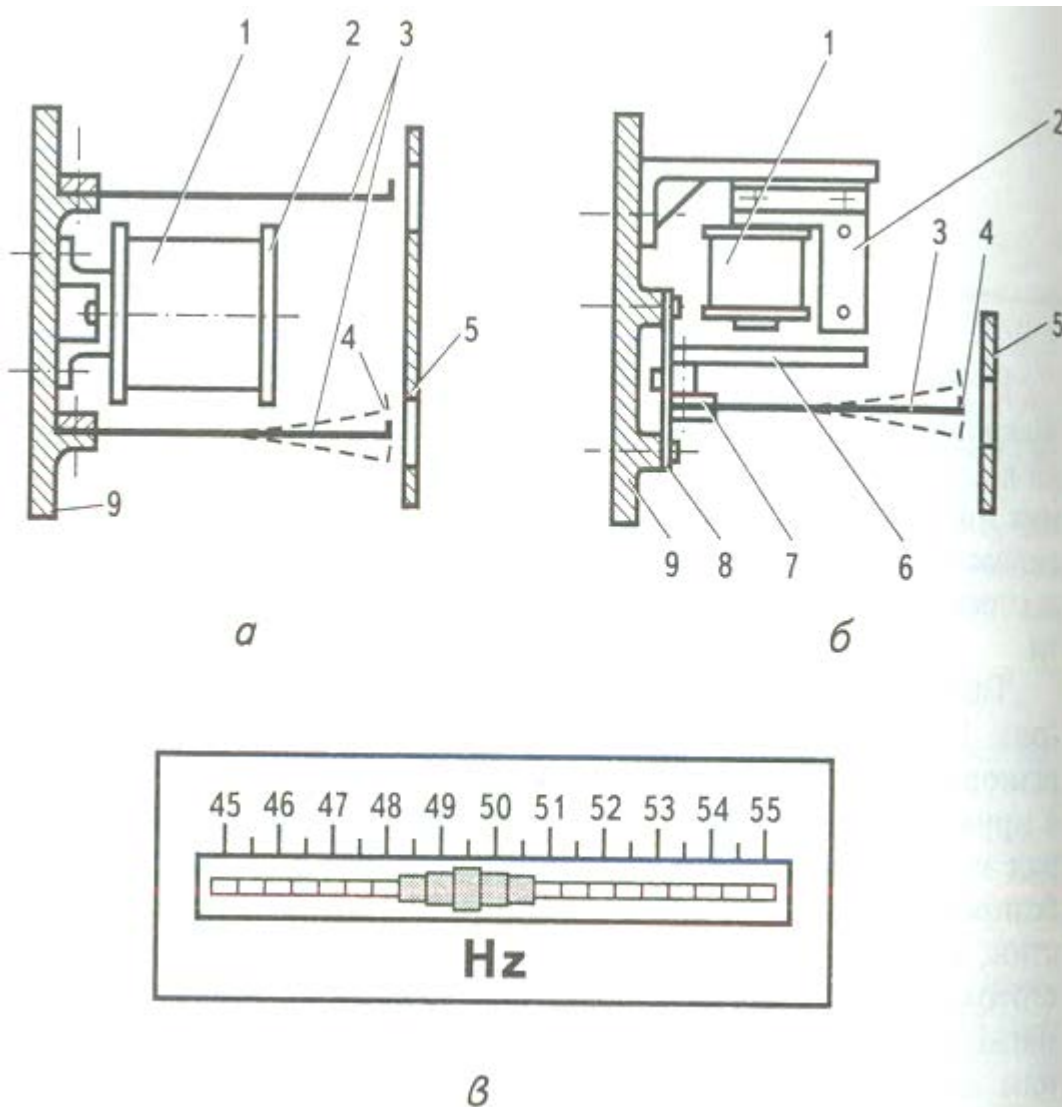
Рисунок 1. Будова вібраційних частотомірів
