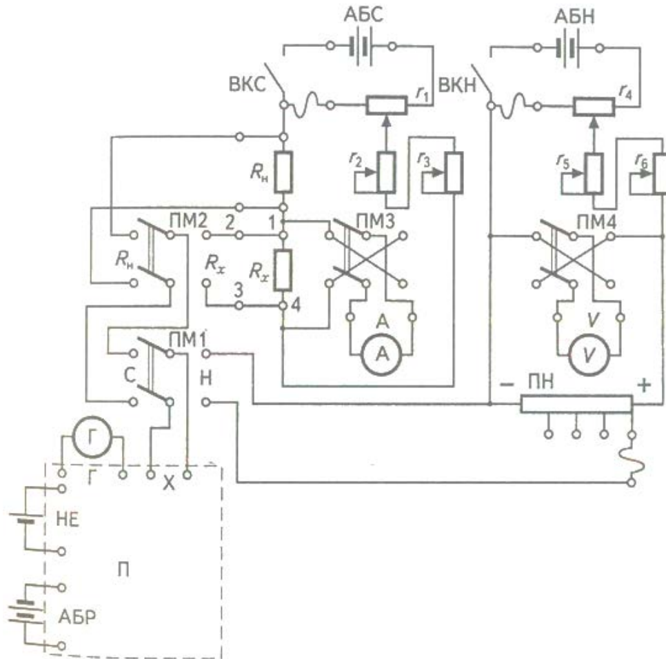
Рисунок 3. Схема для вимірювання величин напруги, струму та опору потенціометром постійного струму
