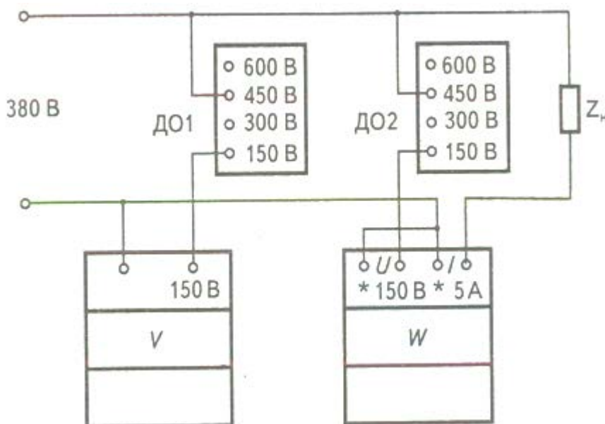
Рисунок 4. Схема вмикання приладів з додатковими опорами
