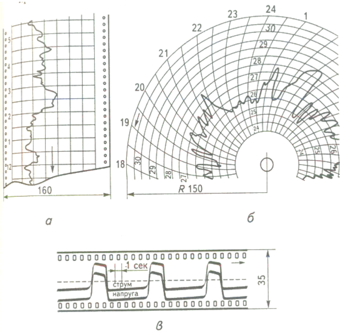
Рисунок 1. Види запису на реєстру вальних приладах: а – на паперовій стрічці; б – на паперовому диску; в – на фотоплівці чи фотопапері
