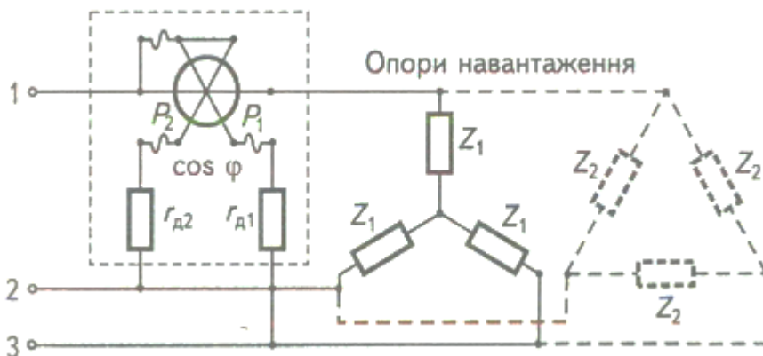
Рисунок 4. Схема ввімкнення фазометра для вимірювання коефіцієнта потужності у трифазному симетричному колі
