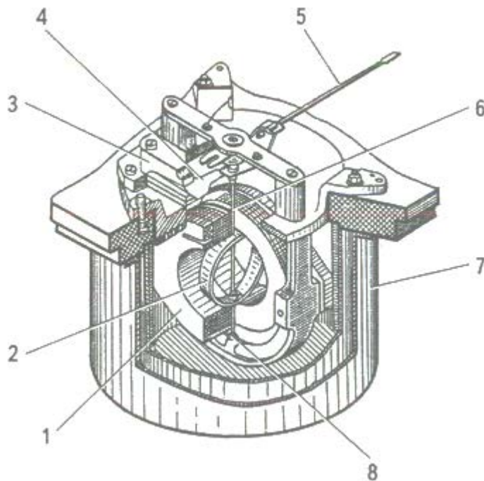
Рисунок 3. Вимірювальний механізм електродинамічної системи
