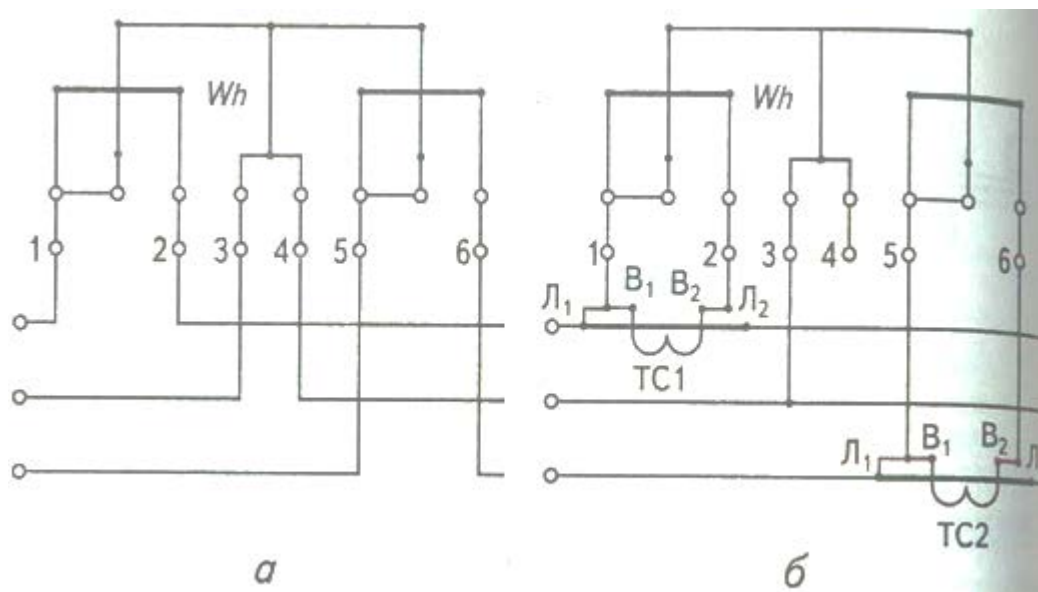
Рисунок 4. Схеми вмикання трифазних двохелементних лічильників: а – пряме; б – за допомогою вимірювальних трансформаторів струму
