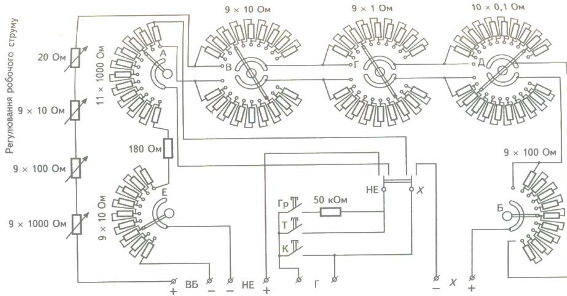
Рисунок 2. Схема потенціометра великого опору
