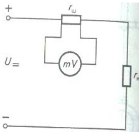
Рисунок 3. Схема вмикання мілівольтметра з шунтом для вимірювання струму
