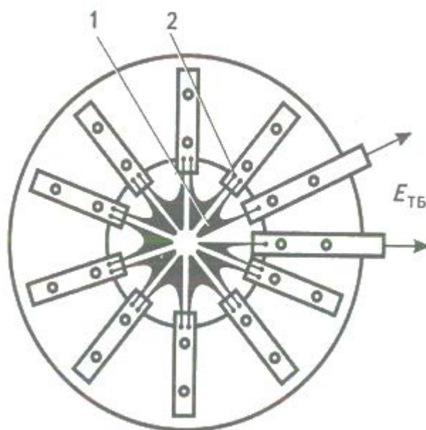
Рисунок 6. Термобатарея радіаційного пірометра
