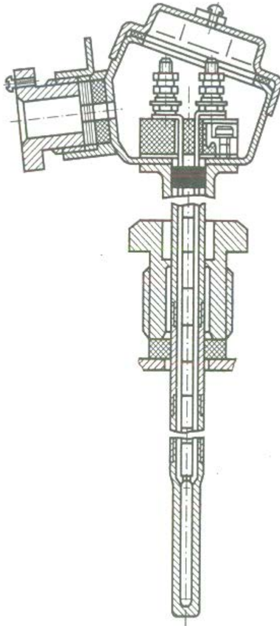
Рисунок 8. Загальний вигляд терморезистора
