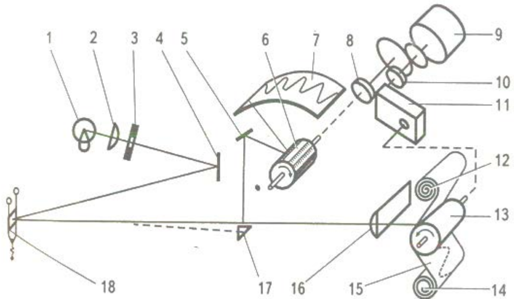
Рисунок 6. Будова електромеханічного осцилографа
