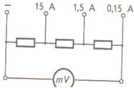
Рисунок 2. Схема універсального шунта з приєднаним до нього мілівольтметром
