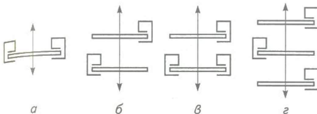
Рисунок 3. Схеми будови трифазних лічильників: a – однодисковий, двохелементний; б – дводисковий, двохелементний; в – дводисковий, трьохелементний; г – тридисковий, трьохелементний
