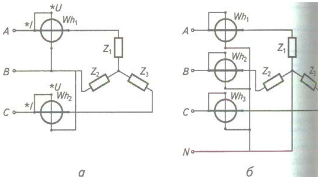
Рисунок 6. Схеми для вимірювання енергії у трифазному колі однофазними лічильниками: а – дволічильникова; б – трилічильникова
