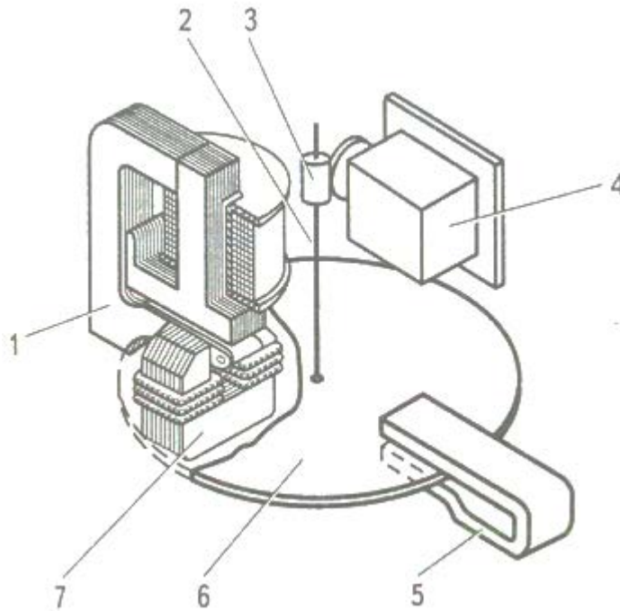
Рисунок 1. Індукційний лічильник електричної енергії однофазного змінного струму
