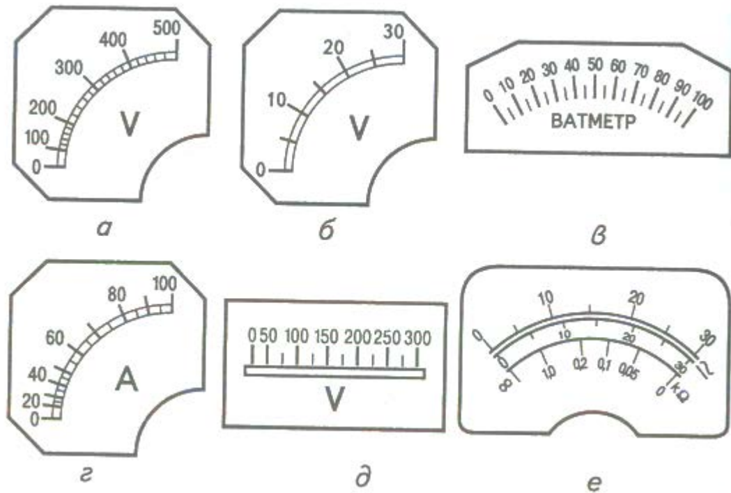
Рисунок 1.2. Шкали електровимірювальних приладів
