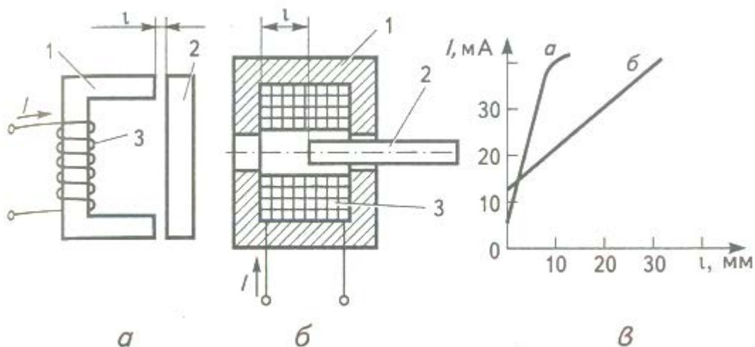
Рисунок 3. Індуктивні перетворювачі
