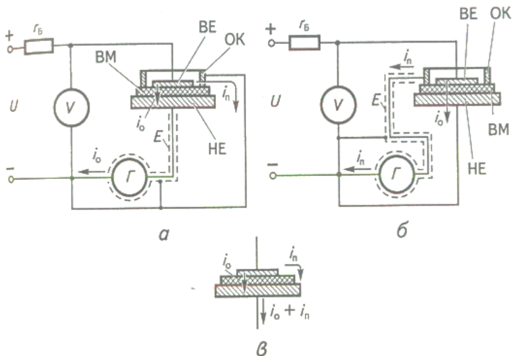
Рисунок 8. Схеми для вимірювання об'ємного та поверхневого опорів ізоляційних металів
