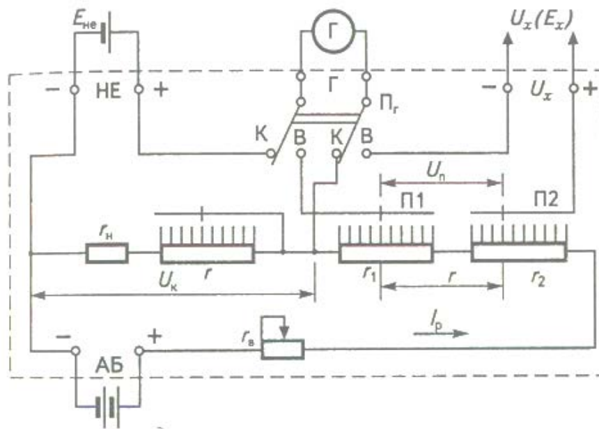
Рисунок 1. Принципова схема потенціометра постійного струму
