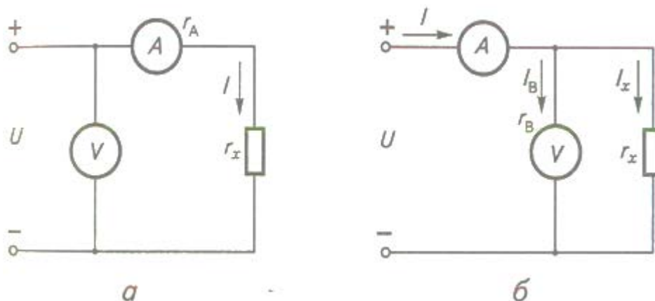
Рисунок 9. Схема для визначення величин опору з допомогою амперметра і вольтметра
