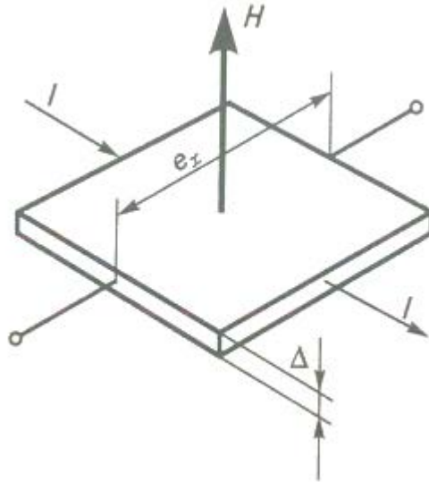
Рисунок 4. Датчик Холла для вимірювання величини напруженості магнітного поля
