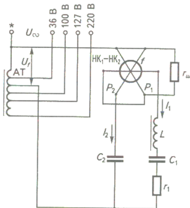
Рисунок 2. Схема електродинамічного частотоміра
