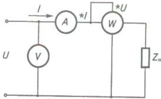
Рисунок 3. Схема вмикання електровимірювальних приладів для посереднього визначення величин коефіцієнта потужності
