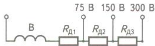
Рисунок 4. Схема триграничного вольтметра
