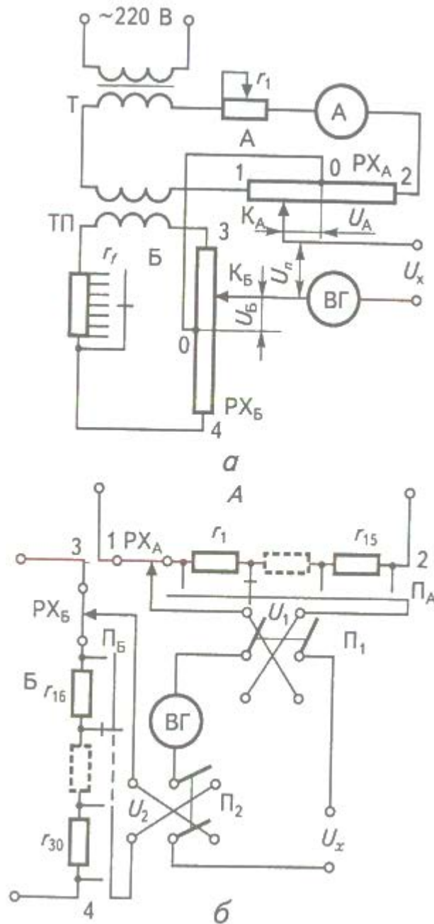
Рисунок 4. Схема потенціометра змінного струму:
