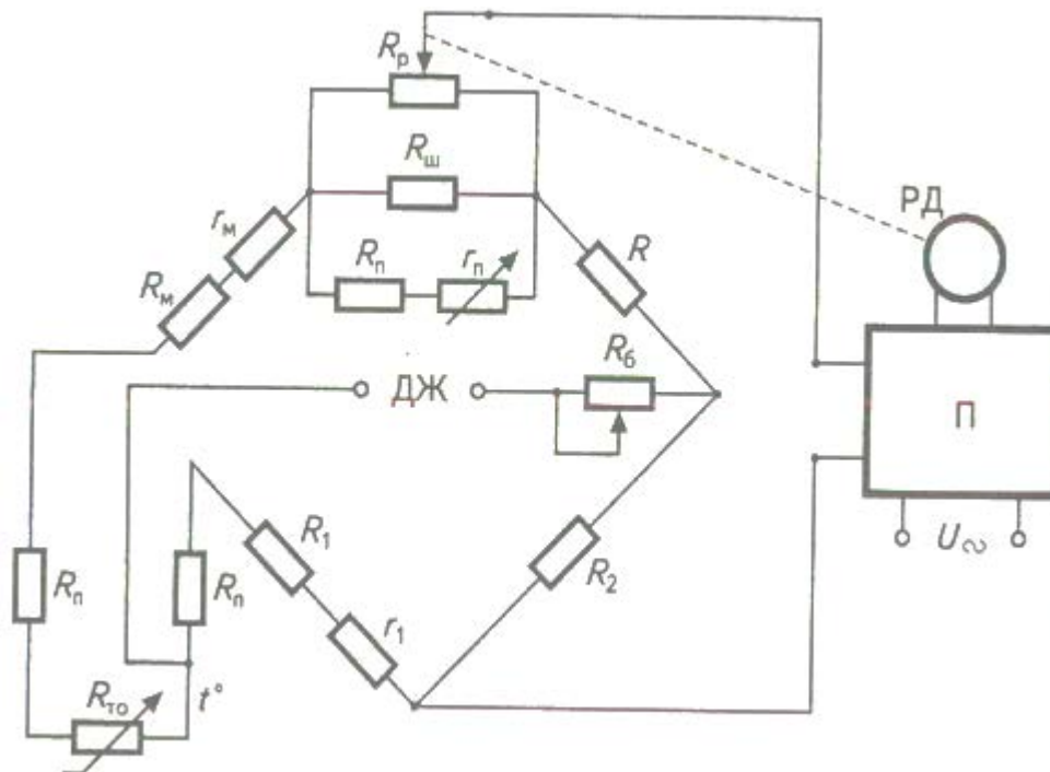
Рисунок 2. Принципова схема автоматичного врівноваженого мосту
