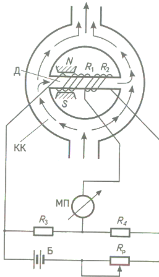
Рисунок 2. Схема термомагнітного газоаналізатора
