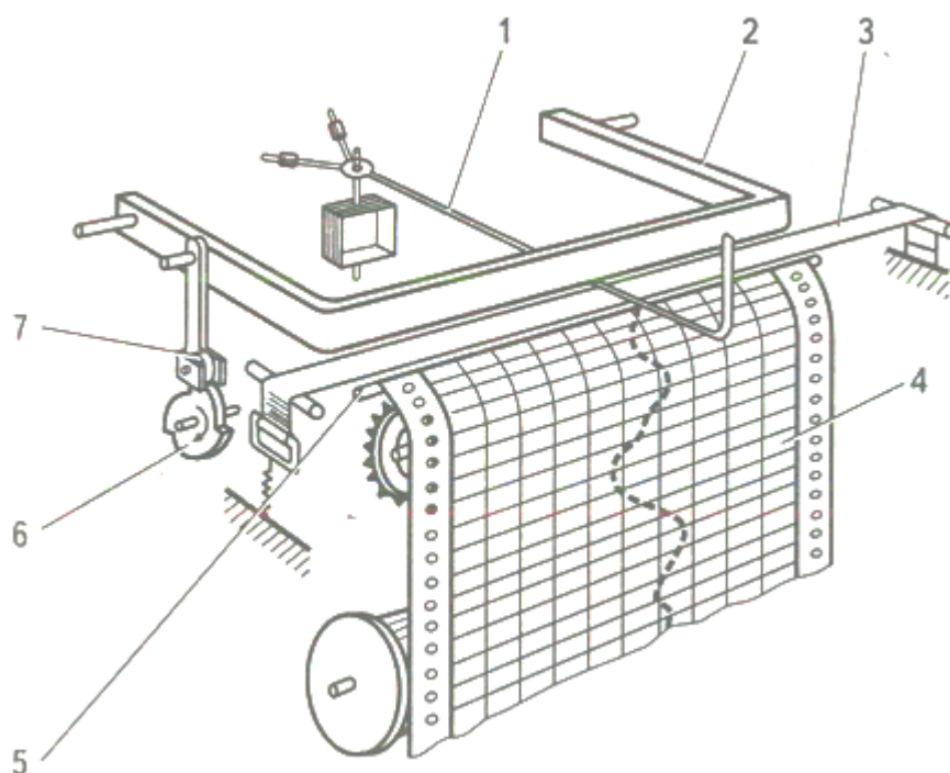
Рисунок 3. Друкувальний пристрій реєстру вального приладу з точковим записом
