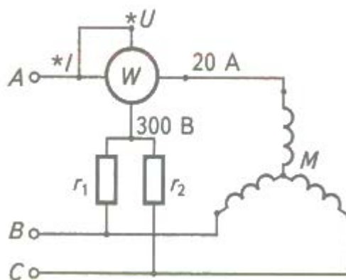
Рисунок 8. Схема вимірювання потужності, споживаної трифазним електродвигуном, однофазним ватметром зі штучною нульовою точкою
