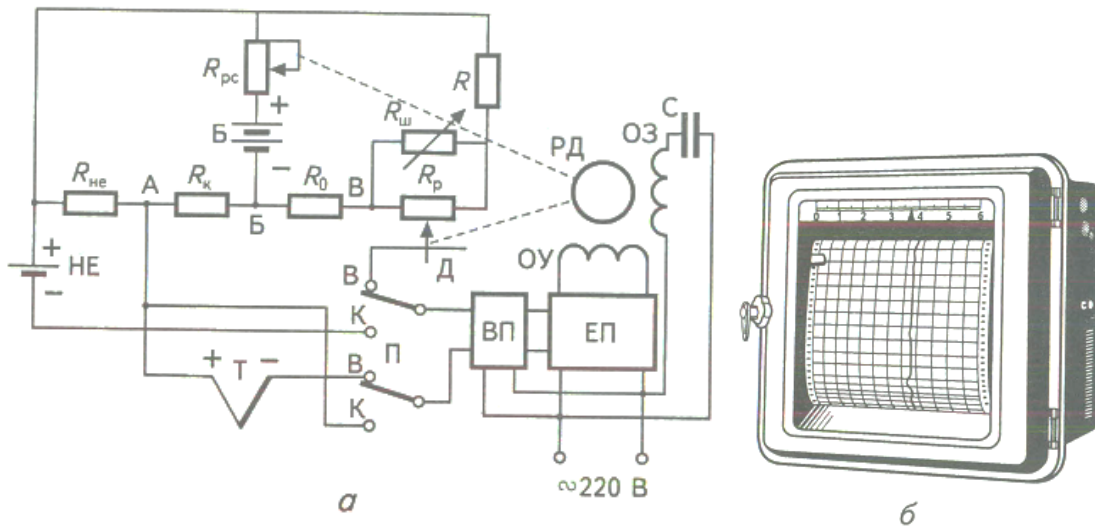
Рисунок 4. Електронний автоматичний потенціометр: а – принципова схема; б – загальний вигляд
