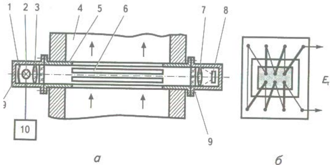
Рисунок 1. Димомір: а – будова; б – термобатарей
