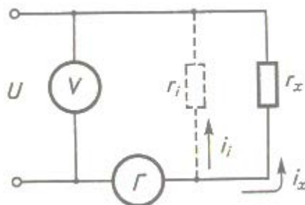
Рисунок 7. Схема, що пояснює вплив опору ізоляції провідників на вимірювання опору значної величини
