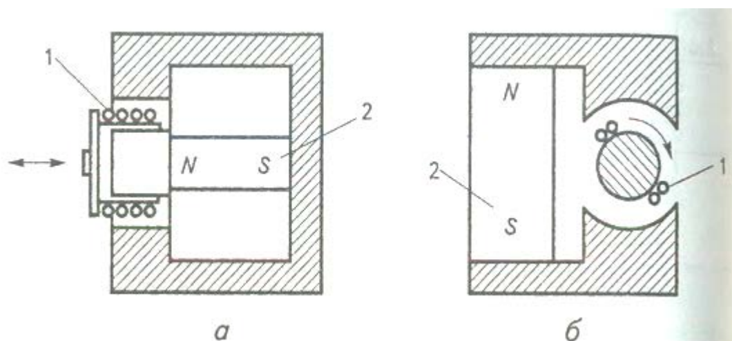
Рисунок 4. Індукційні перетворювачі
