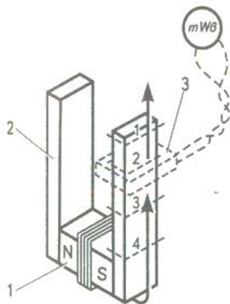
Рисунок 1. Вимірювання величини магнітного потоку постійного магніту флюксометром
