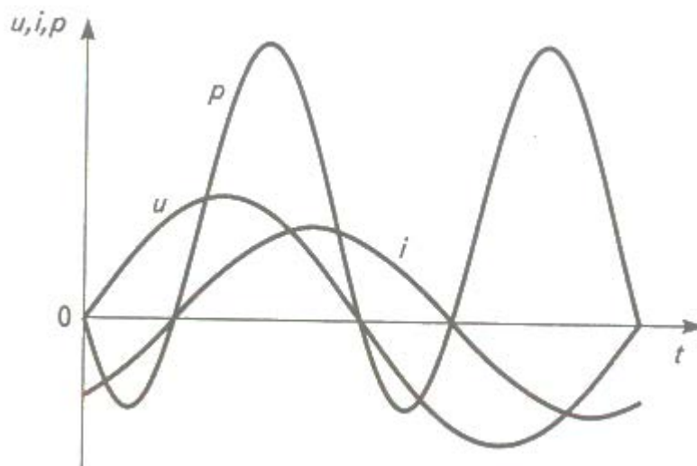
Рисунок 8. Запис величини потужності на змінному струмі
