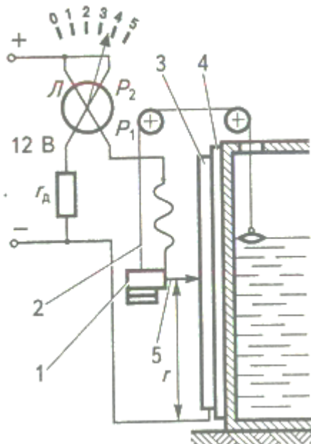
Рисунок 2. Поплавцевий рівнемір з реостатним перетворювачем
