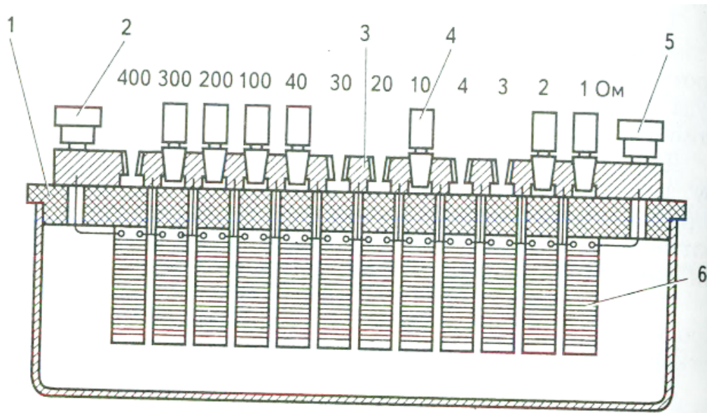
Рисунок 3.3. Штепсельний магазин опорів
