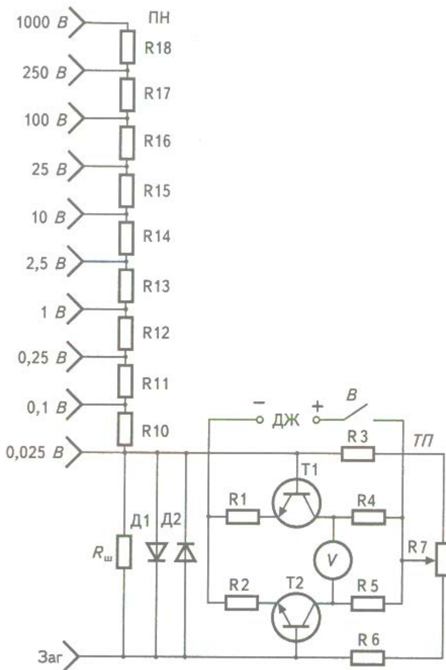
Рисунок 5.1. Схема електронного вольтметра постійного струму на біполярних транзисторах
