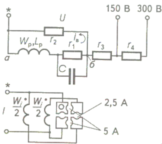
Рисунок 2. Схема переносного ватметра
