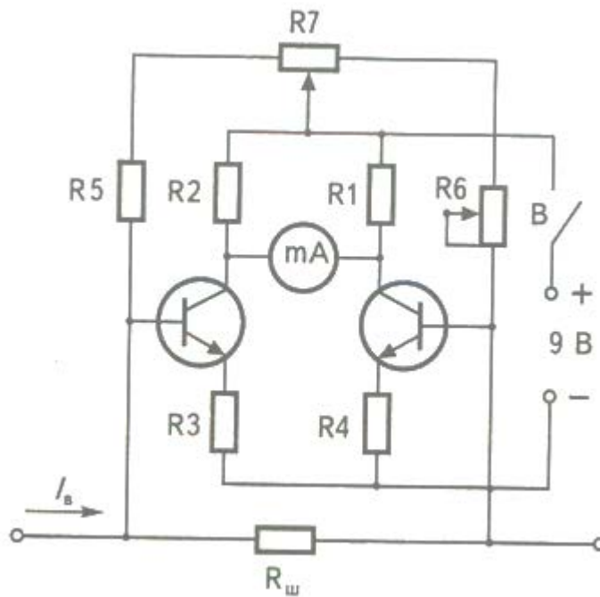
Рисунок 5.3. Схема електронного мікроампер метра
