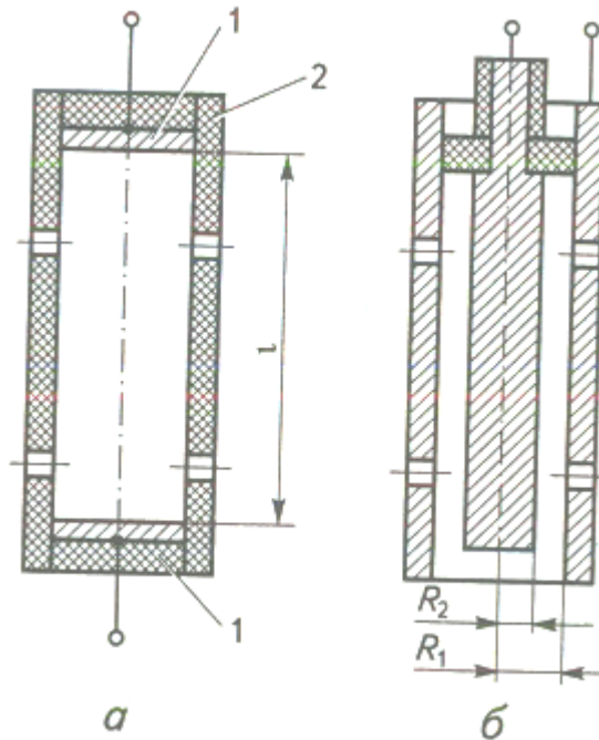
Рисунок 9. Резистивні електролітичні перетворювачі: а – з плоскими електродами; б – з циліндричними електродами
