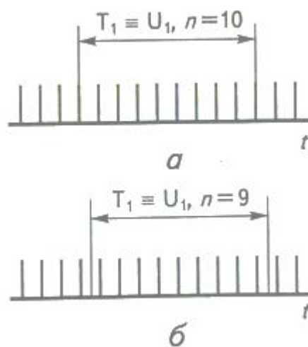
Рисунок 3. Етюри напруг, що показують причину виникнення похибки від дискретності вимірів
