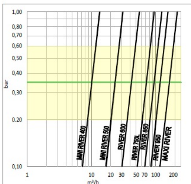
PERDITE DI CARICO IN ZONA DI LAVORO SERIE RIVER / D4.15-0,25 (FLOW RESISTANCE IN WORK AREA RIVER SERIES / D4.15-0,25)
