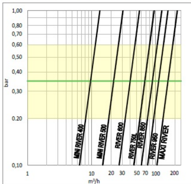
PERDITE DI CARICO IN ZONA DI LAVORO SERIE RIVER / T-0,5 (FLOW RESISTANCE IN WORK AREA RIVER SERIES / T-0,5)
