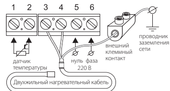
Схема подключения к 3-х проводной электрической сети
