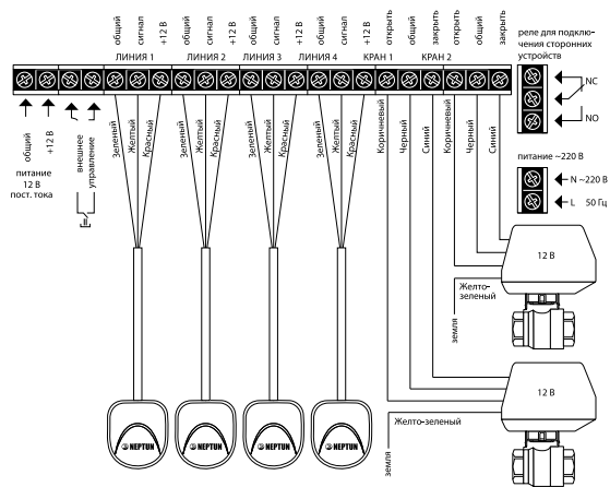
Рис. 4. Схема подключения кранов шаровых с электроприбором DePaLa 12 В к модулю управления Neptun ProW
