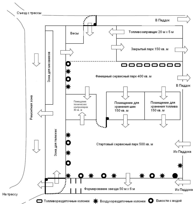
Рисунок 8 - Рекомендуемая планировка сервисного и закрытого парка
