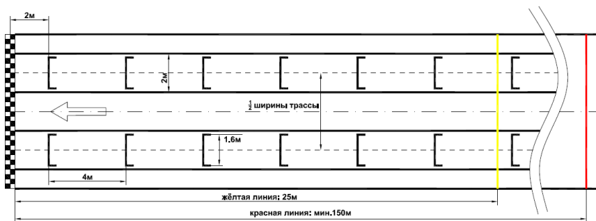
Рисунок 9 - Разметка стартовой решётки
