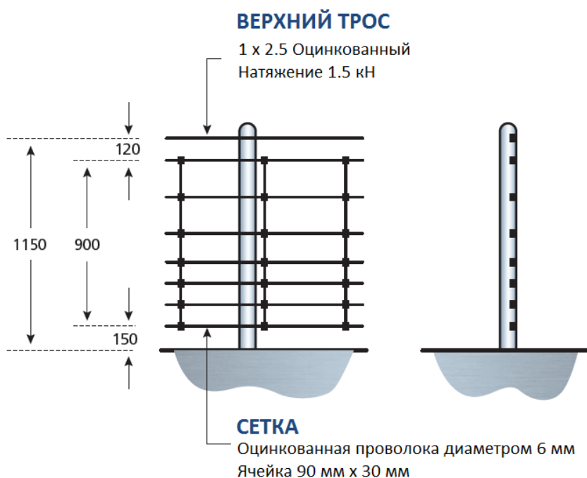
Рисунок 7 - Сетчатое ограждение, допустимо для национальных соревнований
