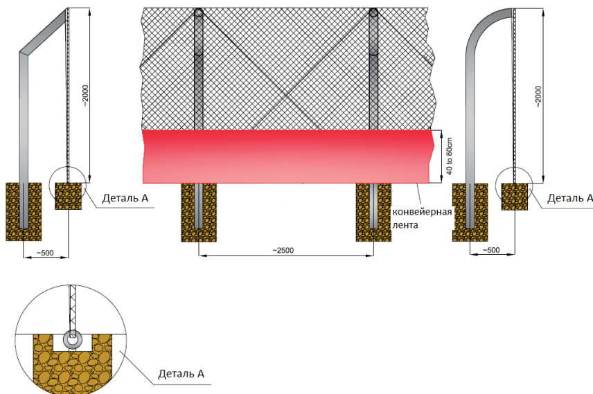
Рисунок 6 – Сетчатое ограждение
