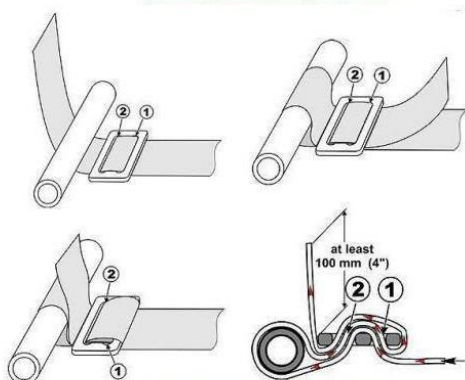
Крепление ремней с "петлевой пряжкой"
