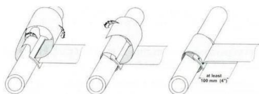
Крепление ремней с "язычком пряжки"
