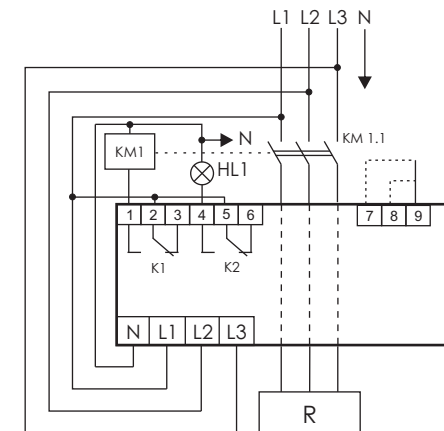
Рис.1 Схема включения с контактором и лампой сигнализации.
