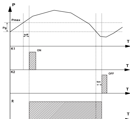
Рис.5 Диаграмма работы.
