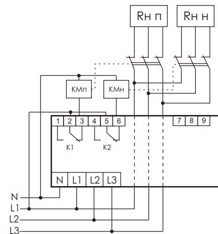
КМп, КМн - контакторы с нормально замкнутыми контактами
