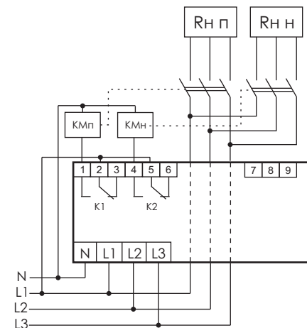
КМп, КМн - контакторы с нормально разомкнутыми контактами
