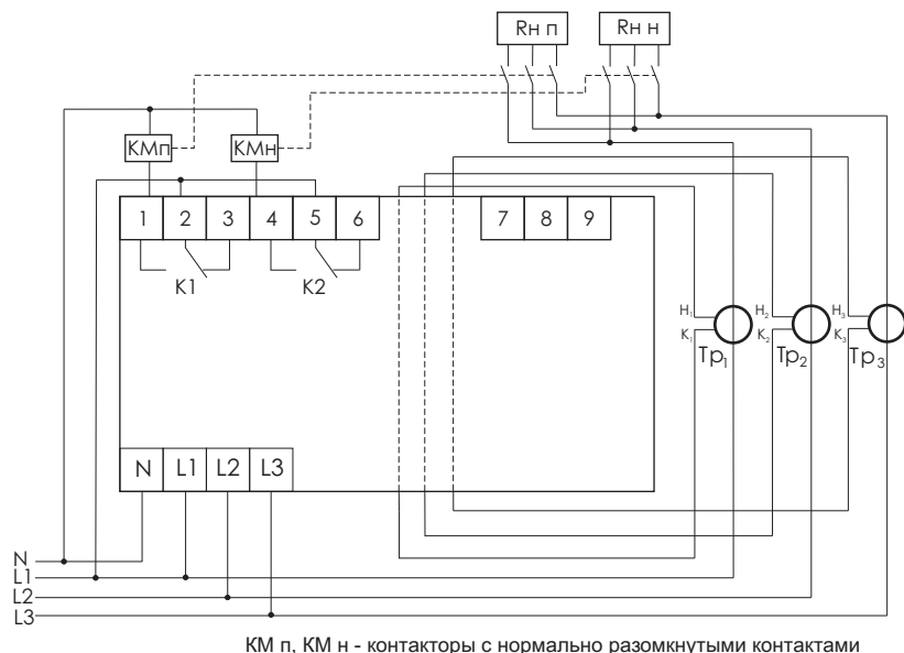
Рис. 8 Схема включения ОМ-630-1 с трансформаторами тока для контроле мощности более 50 кВт.
