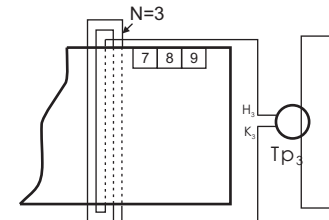
Рис.9 Схема подключения трансформатора тока.
