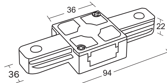
Паспорт изделия
