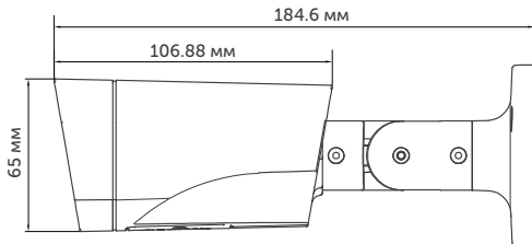
Рис.2 Вид сбоку
