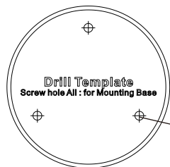
Рисунок 2-4 Шаблон крепления
