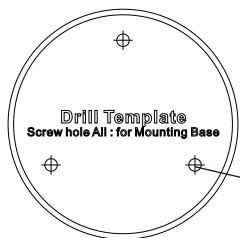
Рисунок 2-1 Шаблон крепления
