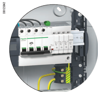
Примечание: для клеммника заземления необходим 1 держатель и 1 комплект клемм
