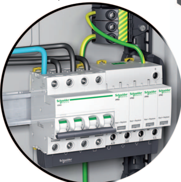
Ограничитель напряжения iPRD 4P + iC60N 4P
