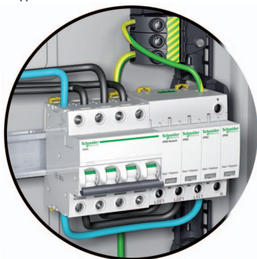
Ограничитель напряжения iPRD 3P+N + iC60N 3P+N
