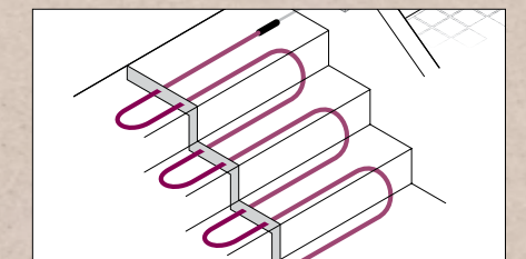
Размещение кабеля на лестнице
