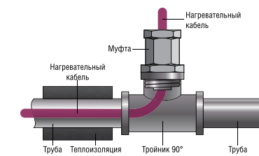
Схема 2. Монтаж муфты в тройник 90^{\circ}
