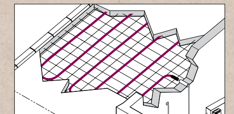
Размещение кабеля на подъездных путях
