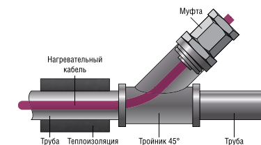
Схема 1. Монтаж муфты в тройник 45^{\circ}
