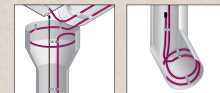
Монтаж кабеля на водосток
