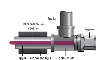
Схема 2. Монтаж муфты в тройник 90^{\circ}
