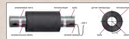
Монтаж кабеля на трубу
