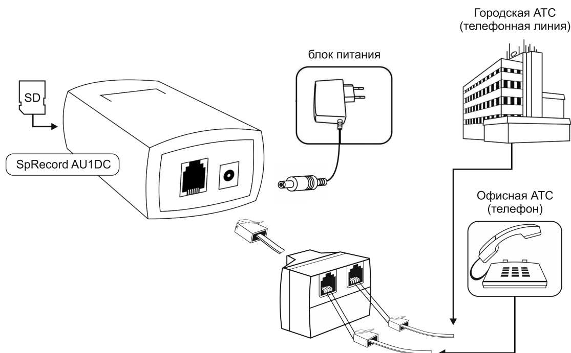
Рисунок 2.1 Схема подключения адаптера SpRecord AU1DC
