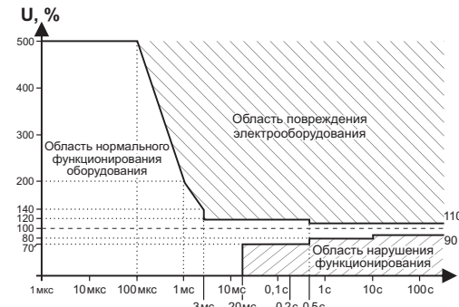
Рисунок 1. Кривая работы электрооборудования ITIC (CBEMA), ( http://www.home.agilent.com/upload/cm_upload/All/1.pdf?&cc=UA&lc=eng ).
