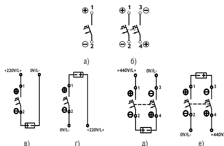
а) однополюсного; б) двухполюсного и примеры подключения в сетях постоянного тока в), г) однополюсного; д), е) двухполюсного Рисунок Г.2 - Принципиальные электрические схемы выключателей постоянного тока
