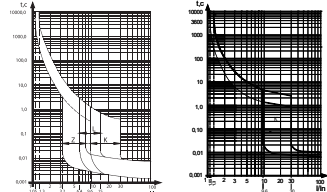
Рисунок Б.4 Защитные характеристики в цепи постоянного тока по ГОСТ Р 50030.2 при контрольной температуре плюс 30°C.
