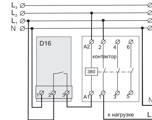
Схема 4. Подключение реле напряжения и контактора с обмоткой 380 VAC
