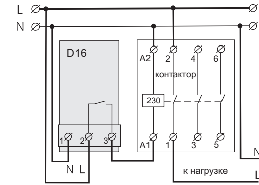
Схема 3. Подключение реле напряжения и контактора с обмоткой 230 VAC
