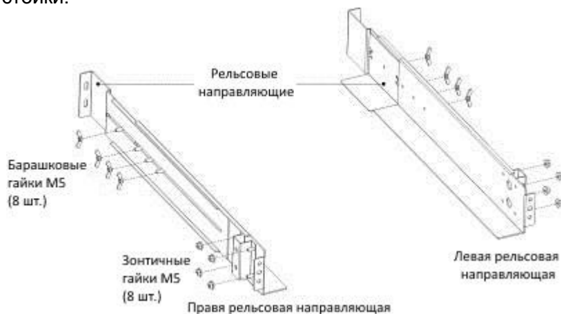
Рис. 4 Крепление рельсовых направляющих
