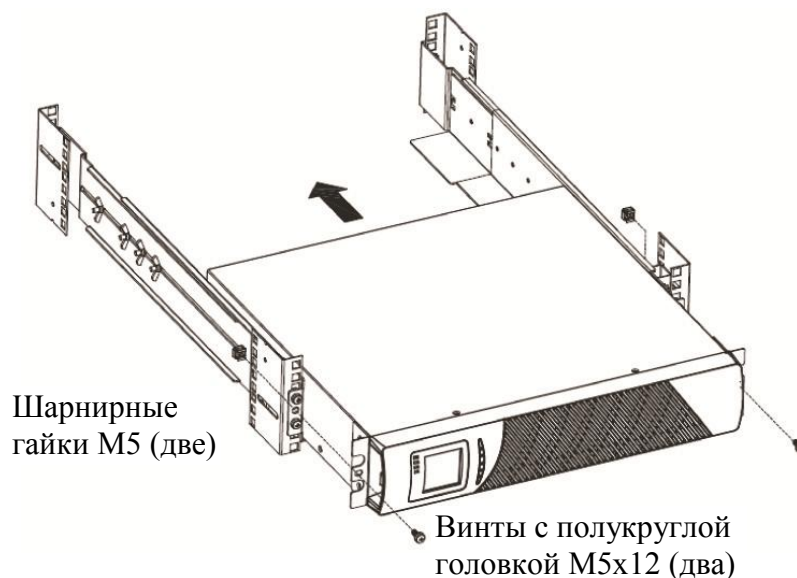
Рис. 7 Фиксация передней части блока ИБП
