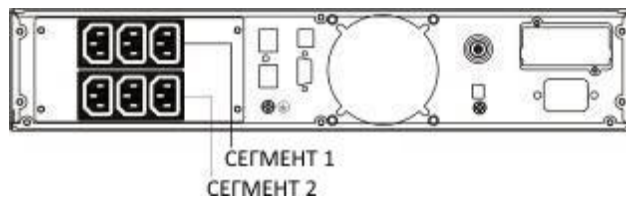
Рисунок 30. 1000 ВА Rack/Tower
