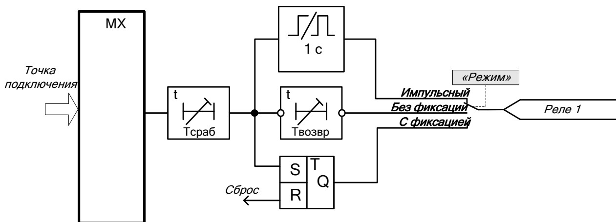
Рисунок 12 – Фрагмент функциональной логической схемы программируемого реле
