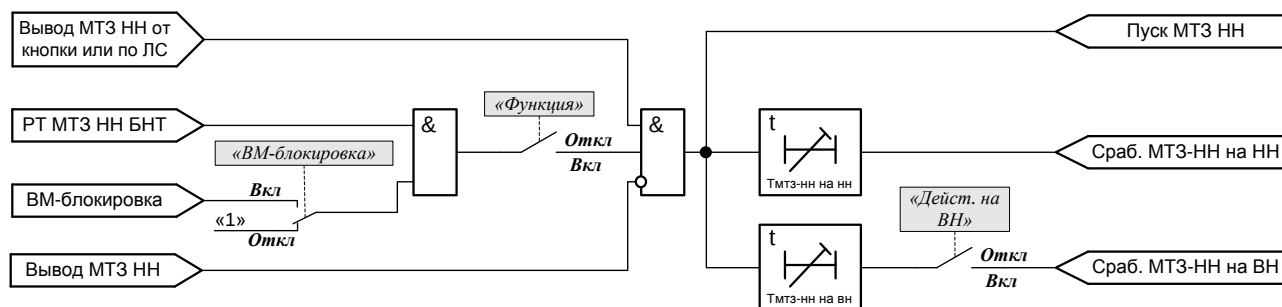
Рисунок 8 – Функционально-логическая схема МТЗ НН
