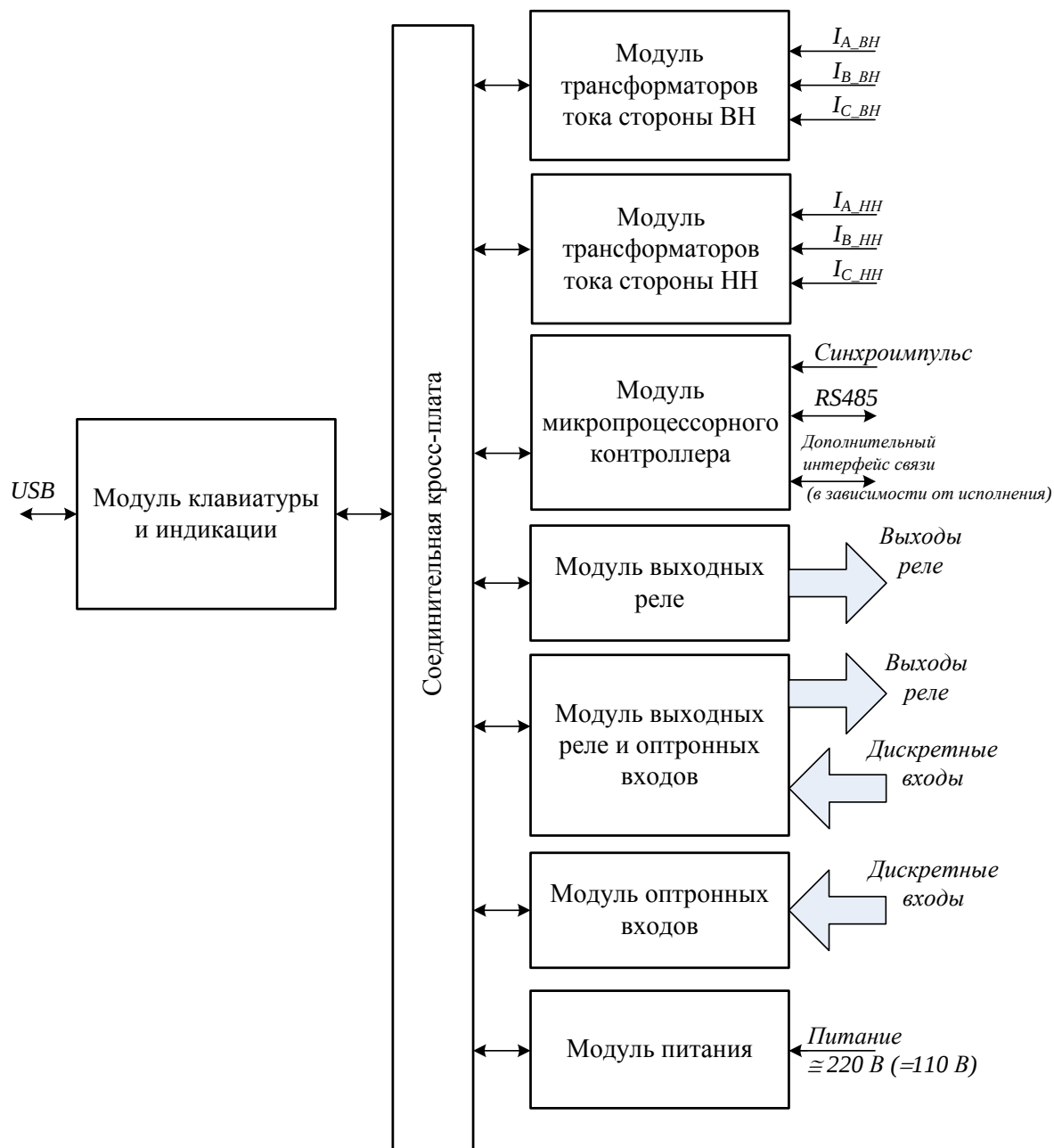
Рисунок 13 – Структурная схема устройства «Сириус-Т»
