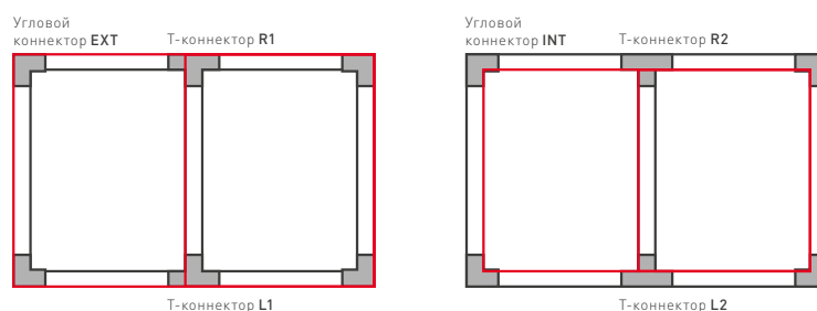
Рисунок 2. Выбор коннектора исходя из расположения заземляющего контакта на шинопроводе
