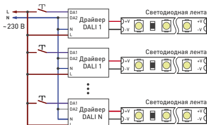
Рисунок 4. Схема подключения нескольких источников питания при использовании управления Push Dim.
