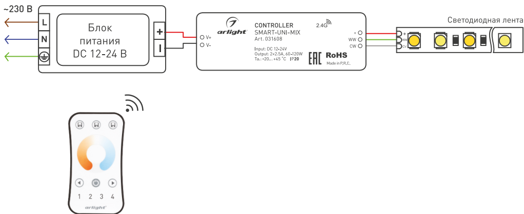
Рисунок 1. Схема подключения контроллера SMART-UNI-MIX
