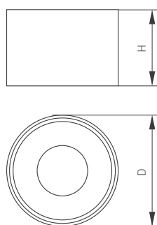
Рис. 1. Чертеж и габаритные размеры
