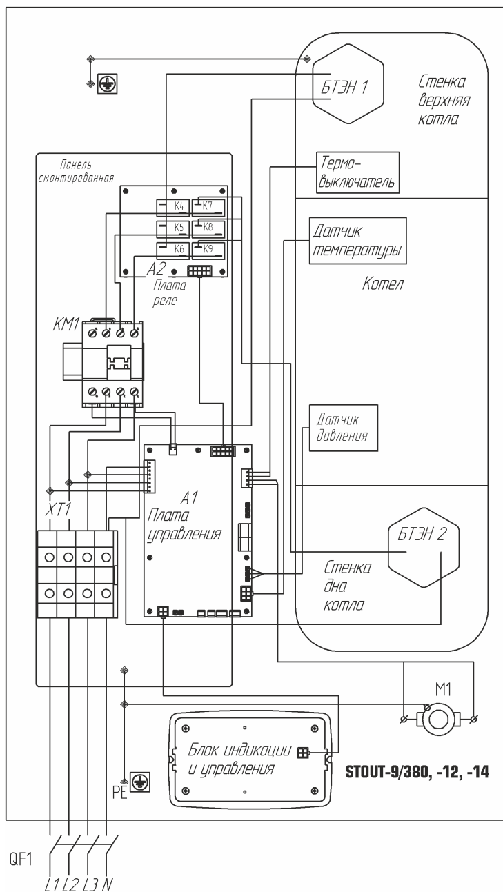
Рисунок 14 Схема подключения SEB-0001-000009÷SEB-0001-000014 к сети 380 В.
