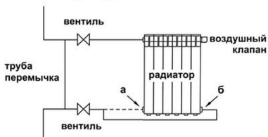
однотрубная система
