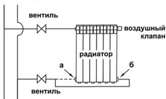
двухтрубная система
