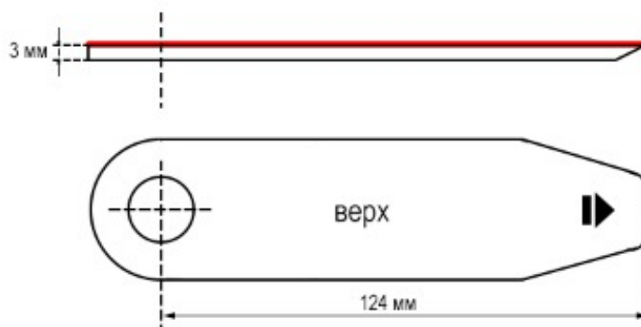
Рис. 1.5 Выносная пластина для измерения наклонной высоты антенны
