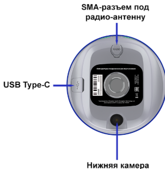
Рис. 1.2 Корпус приёмника PrinCe i20AR
