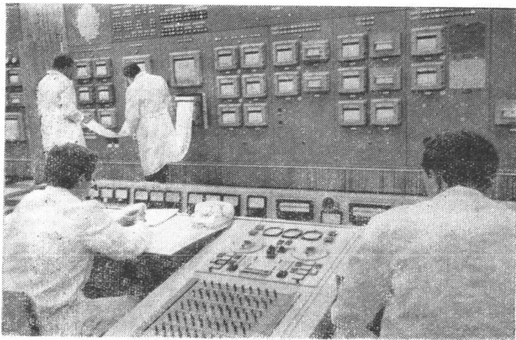
Пульт управления атомным реактором БОР-60.
