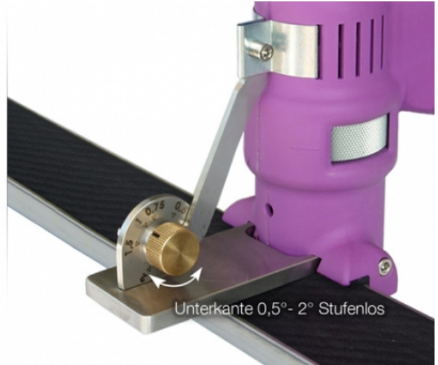
Schleifvorrichtung Unterkante für Disc Man 2 und 4
