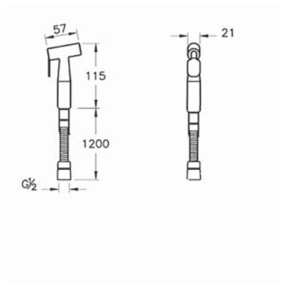
Гигиенический душ
