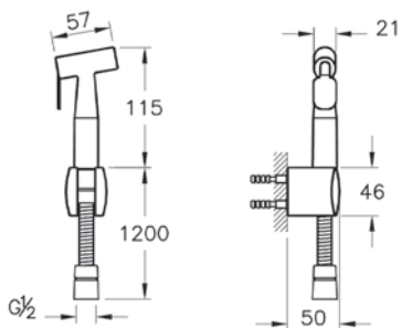
Гигиенический душ
