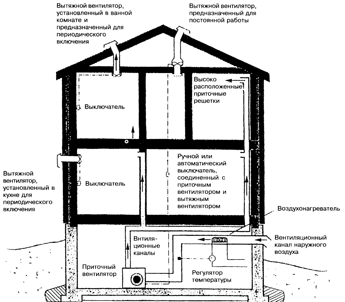
Рисунок 7.2 — Система воздушного отопления с принудительной циркуляцией воздуха, совмещенная с системой механической вентиляции, не присоединенная к системе теплоснабжения
