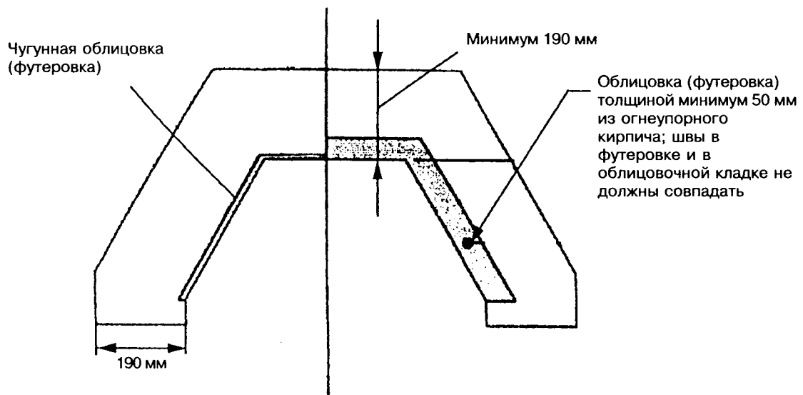
Рисунок 7.5 — Футеровка камина
