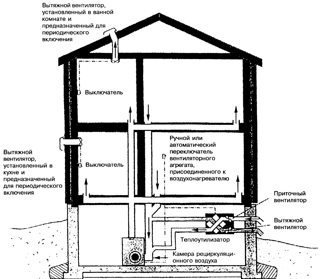
Рисунок 7.3 — Присоединение теплоутилизационного агрегата к камере подогрева воздуха
