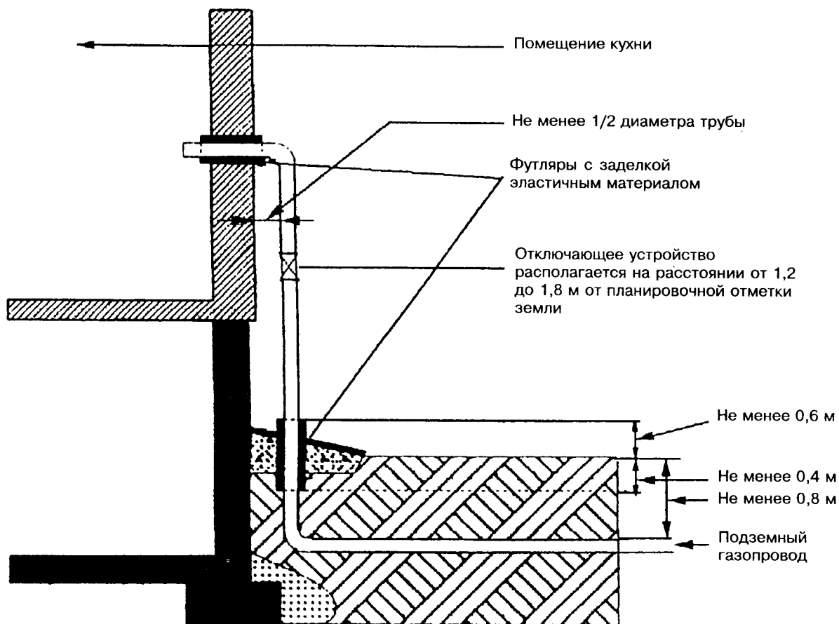
Рисунок 9.1 — Газовый ввод
