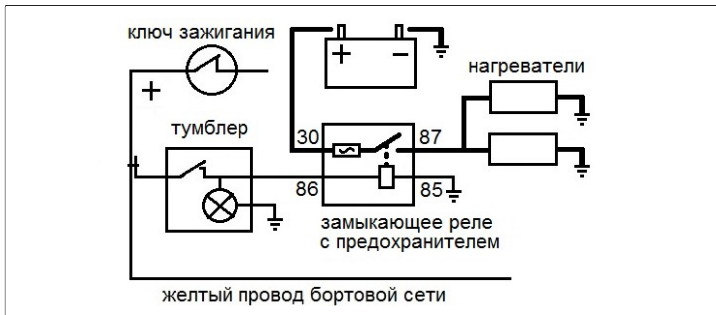
Рис.1. Схема подключения реле управления НАГРЕВАТЕЛЯ
