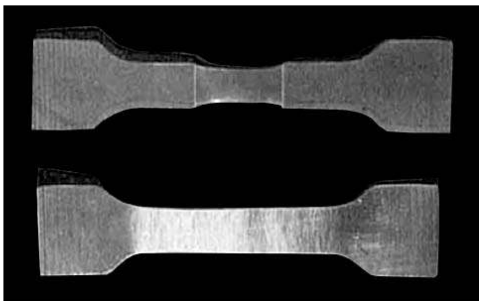
Рис. 2. Внешний вид образцов полиэтилентерефталата, растянутых на воздухе (а) и в адсорбционно-активной среде (н-пропанол) (б).
