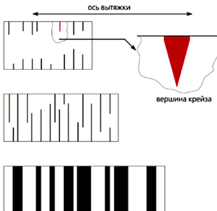
Рис. 4. Схематическое изображение отдельных стадий крейзинга полимера: I - инициирование крейзов, II - рост крейзов, III - уширение крейзов.
