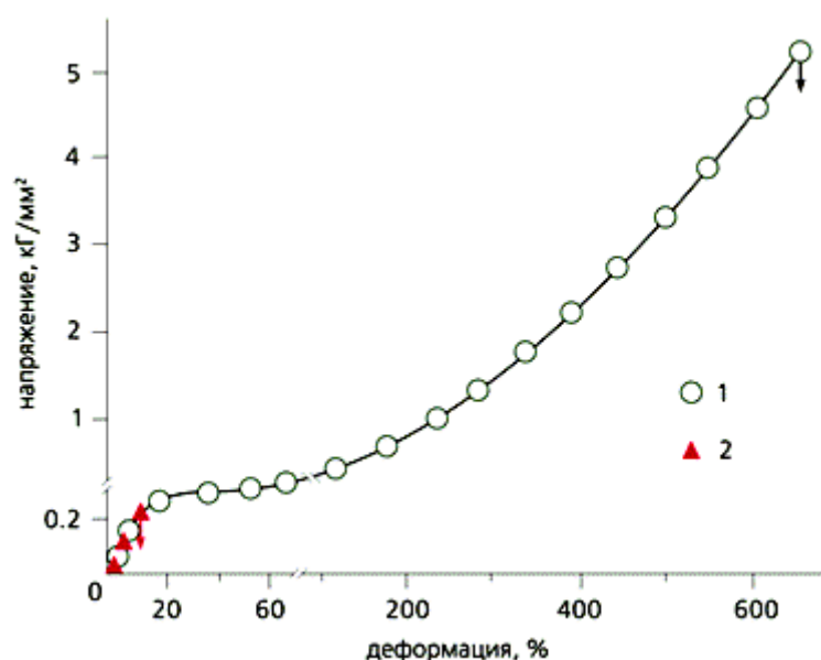
Рис. 1. Зависимость напряжения от деформации монокристаллов цинка при 400°C: 1 - на воздухе; 2 - в расплаве олова.
