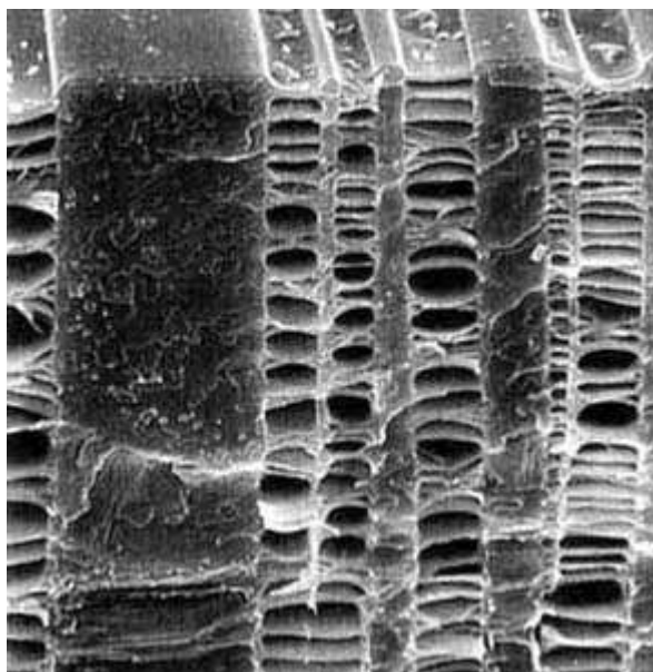
Рис. 3. Электронная микрофотография образца полиэтилентерефталата, деформированного в n-пропанол. (Увел. 1000.)
