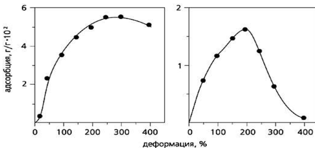
Рис. 7. Зависимость величины адсорбции от степени вытяжки полиэтилентерефталата в n -пропанол: а - водные растворы йода; б - водные растворы родамина С.
