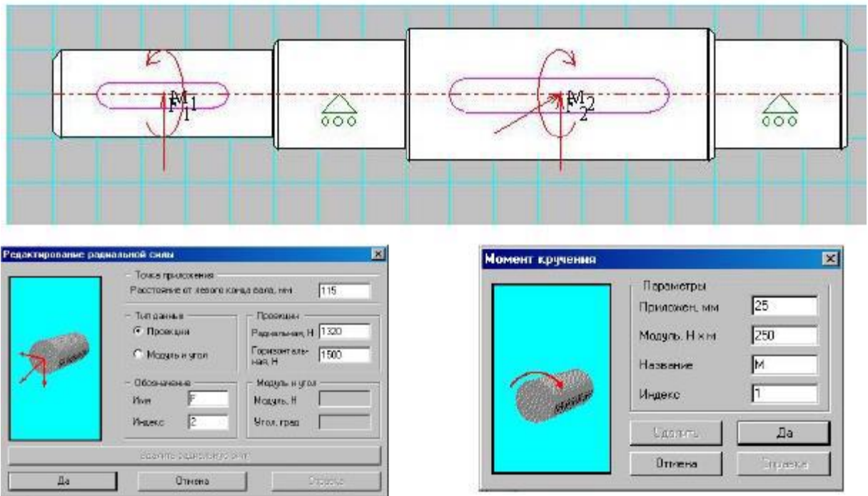
Рисунок 1 – Расчет вала в APM Shaft.
