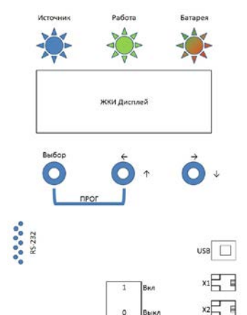
Внешний вид контроллера 60А
