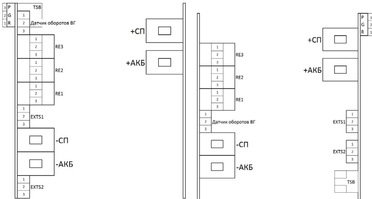
Вид на контакты и разъёмы контроллера 100А
