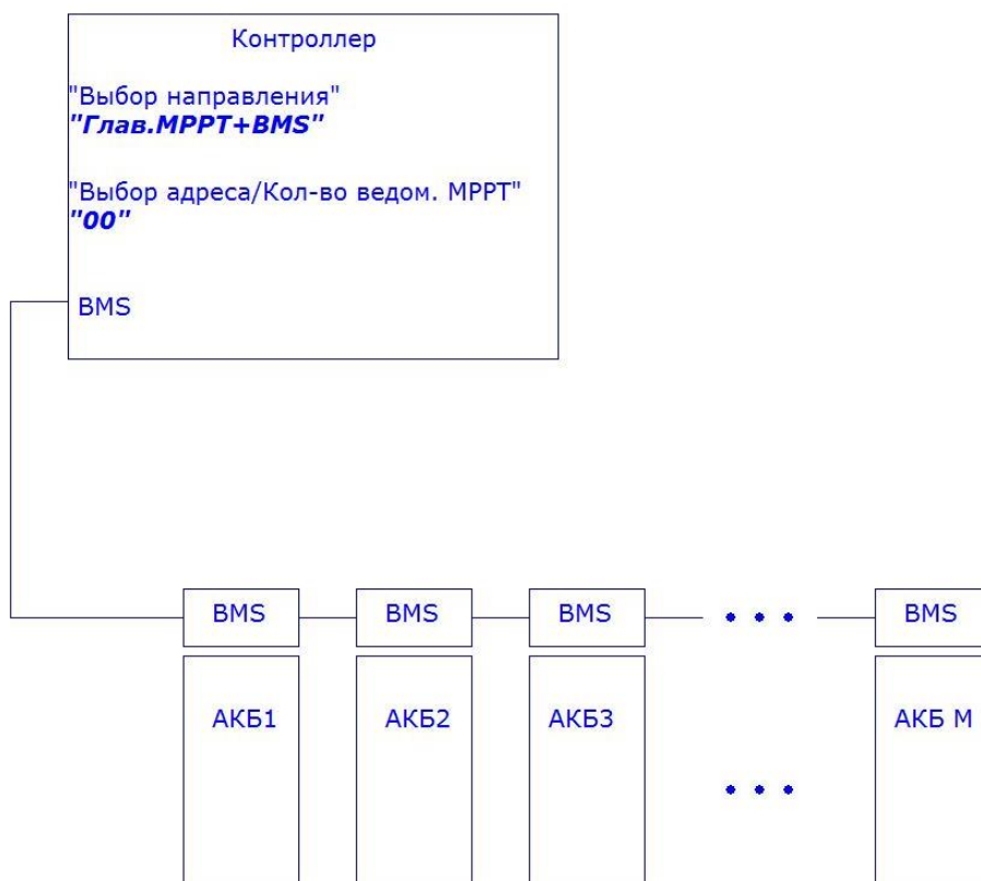
Рис. П10. Схема системы "Контроллер+BMS". Новая версия.
