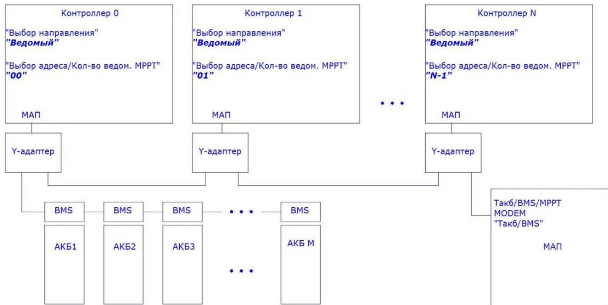
Рис. П2. Схема системы "Несколько Контроллеров+МАП+BMS". Старая версия.
