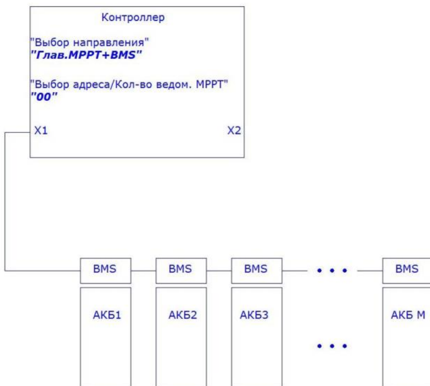
Рис. П9. Схема системы "Контроллер+BMS". Новая версия.
