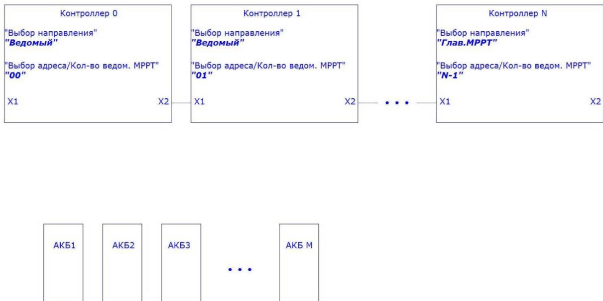
Рис. П7. Схема системы "Несколько Контроллеров". Новая версия.
