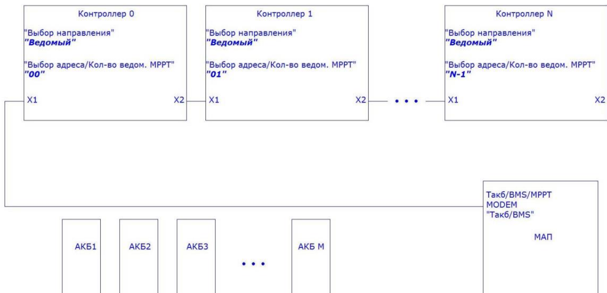
Рис. П3. Схема системы "Несколько Контроллеров+МАП". Новая версия.
