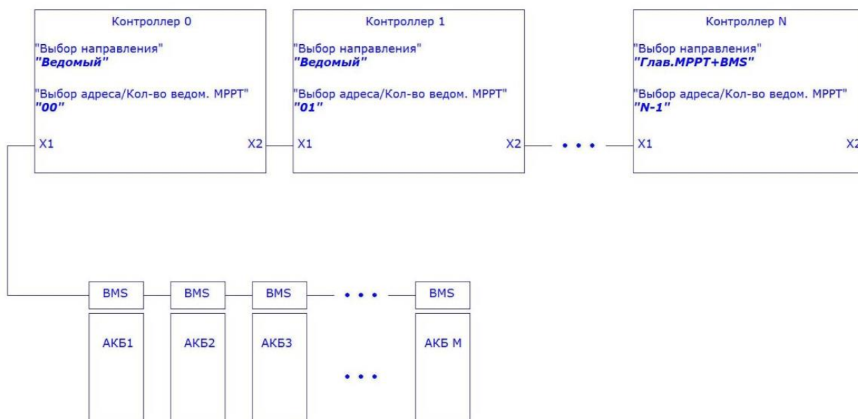
Рис. П5. Схема системы "Несколько Контроллеров+BMS". Новая версия.
