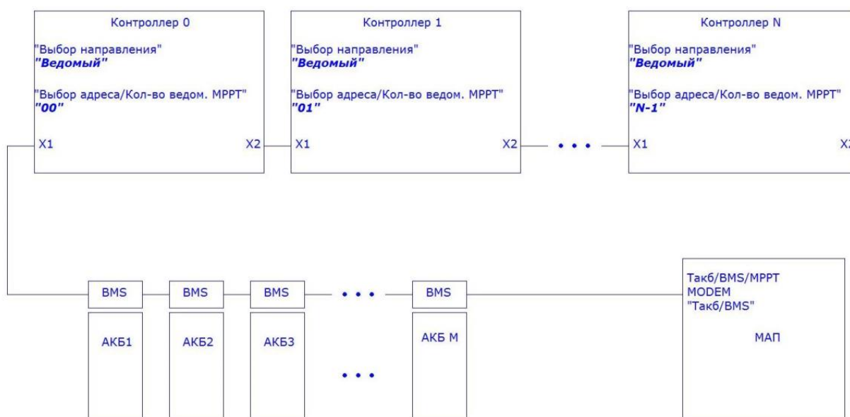
Рис. П1. Схема системы "Несколько Контроллеров+МАП+BMS". Новая версия.
