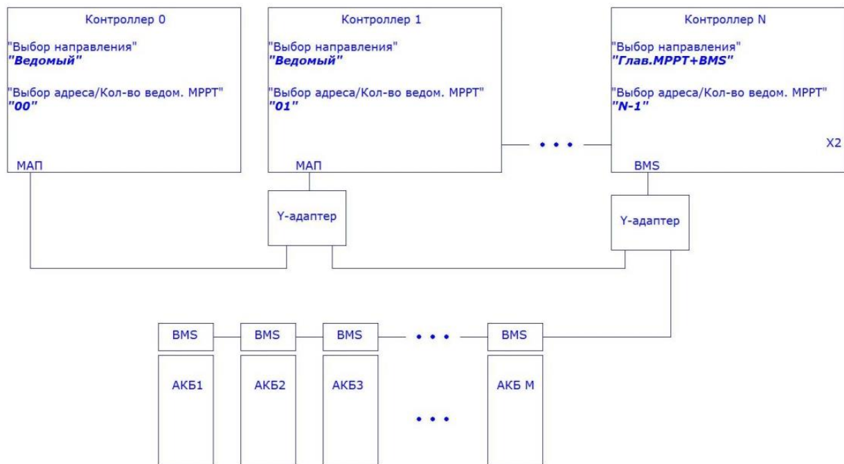
Рис. П6. Схема системы "Несколько Контроллеров+ВМС". Старая версия.
