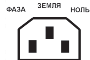
Рисунок 4. Вход сети приборов мощностью до 3 кВт
