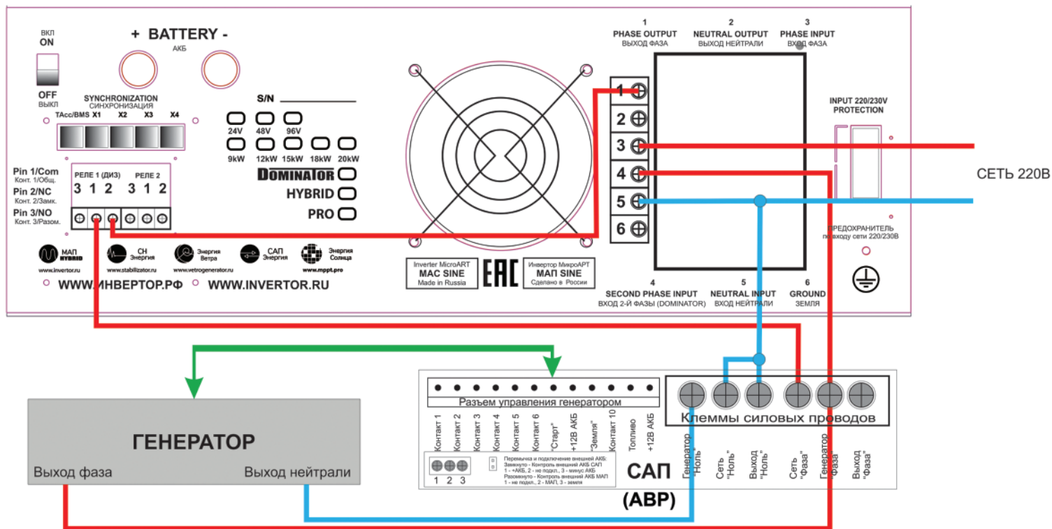
Рисунок 15. Пример подключения Бензо/Газо/Дизель генератора на 2-й вход МАП DOMINATOR с помощью САП или ABP
