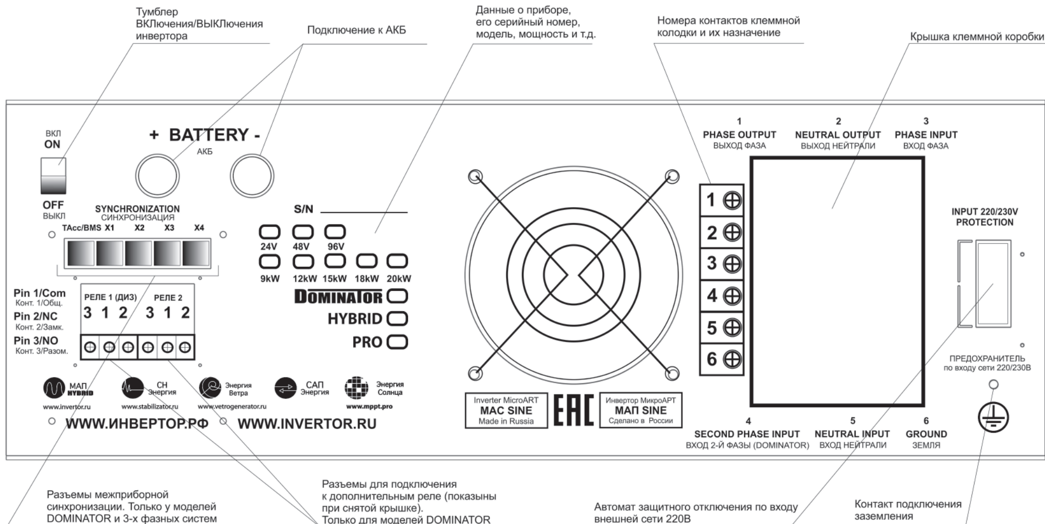
Рисунок 2. Внешний вид инвертора, задняя сторона
