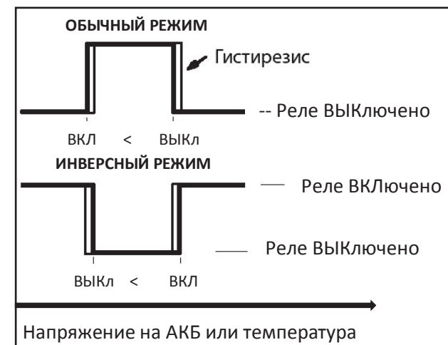
Рисунок 11. Режимы работы Реле
