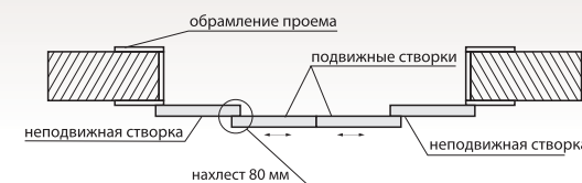
Установка перегородки вне проема
