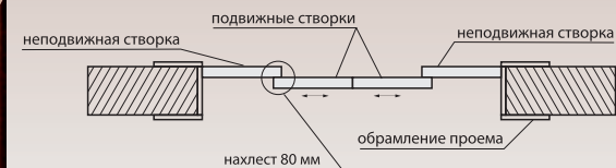
Установка перегородки в проем
