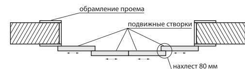
Установка перегородки с четырьмя активными створками
