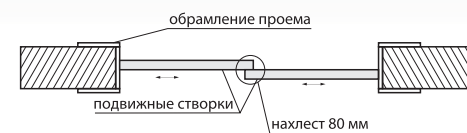
Установка перегородки в проем
