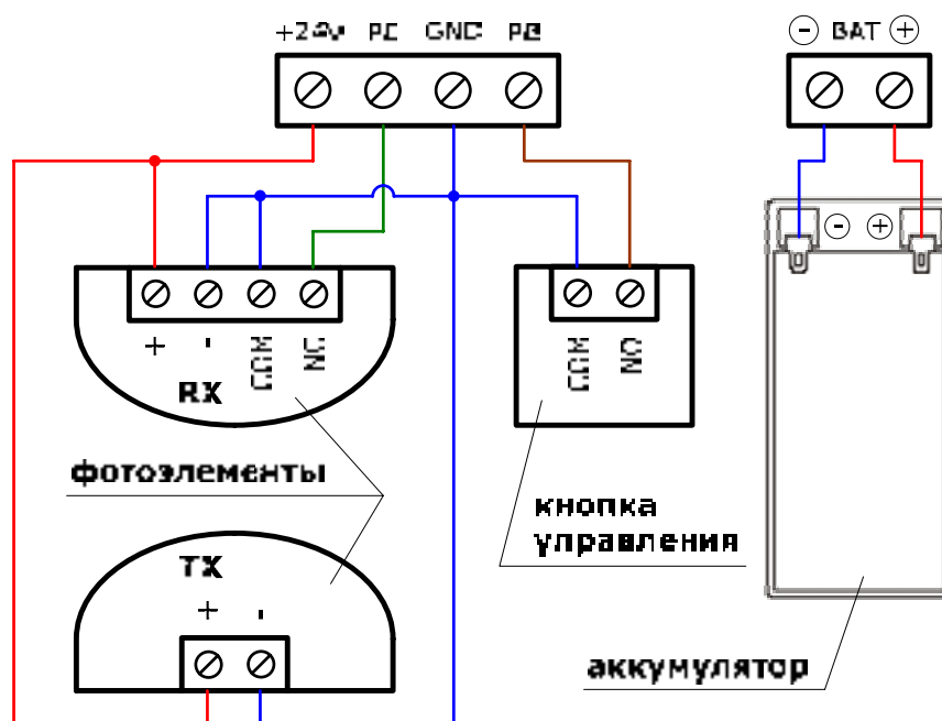
Рис. 4. Электрические подключения
