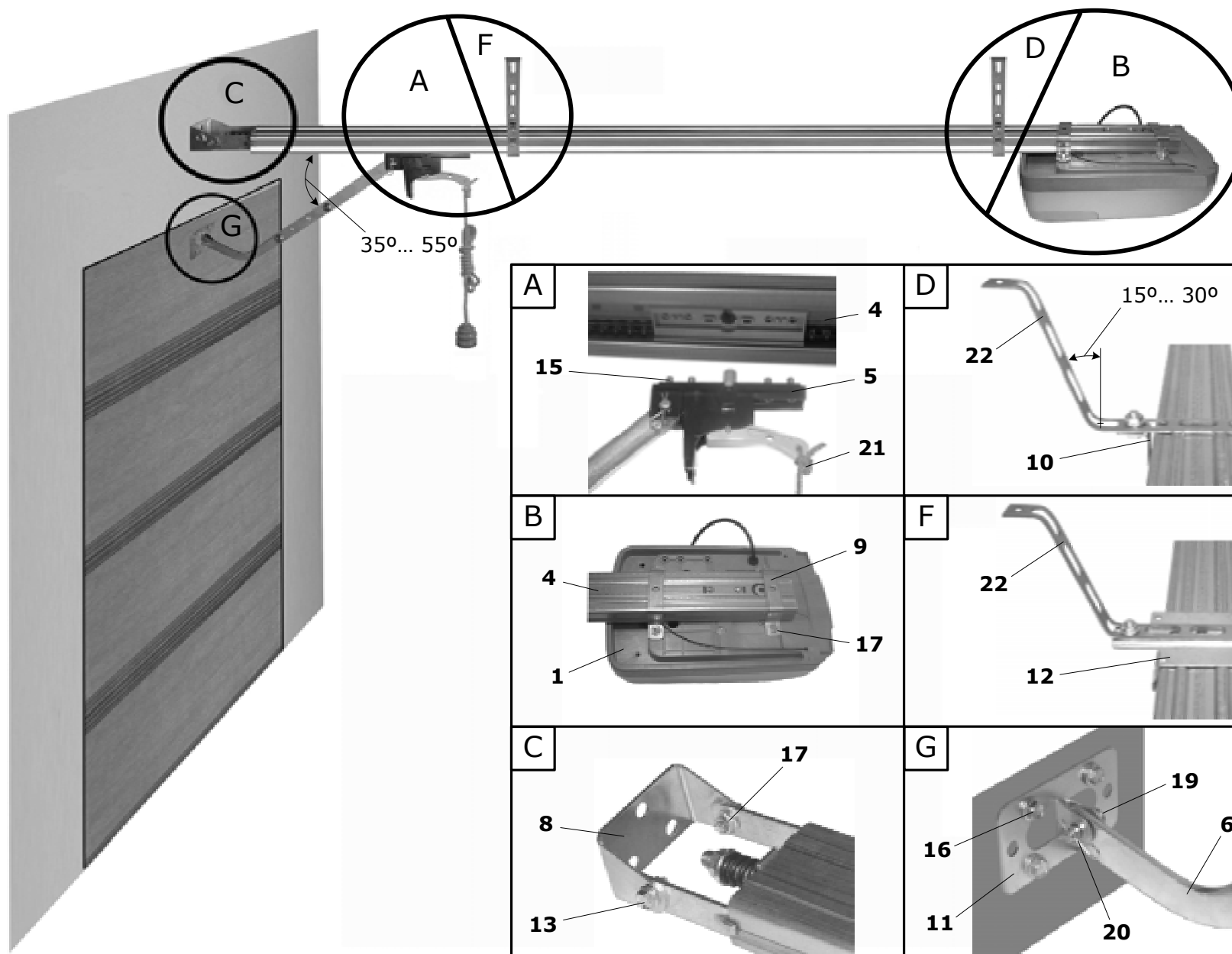
Рис. 2. Монтаж комплекта
