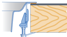
Нержавеющая сталь: установка мойки с плоским кантом поверх столешницы
