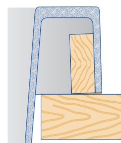
SILGRANIT® PuraDur®: накладной модуль
