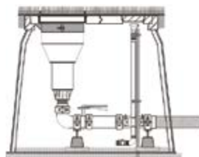
ВИД СБОКУ
