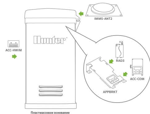
Коммуникационные элементы ACC на пластмассовом основании
