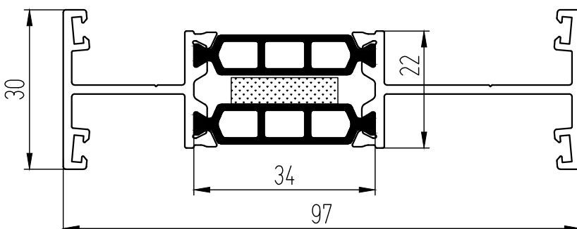
Соединитель рам (комбинированный) с термоизолирующим наполнителем
