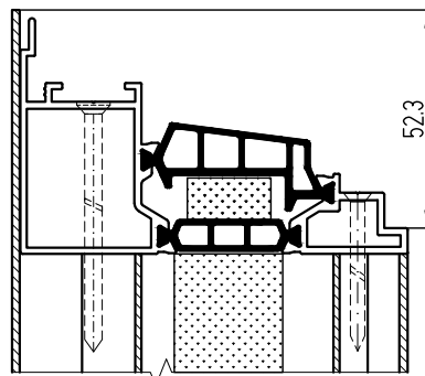
Обработка притвора створки СТ8517Т
