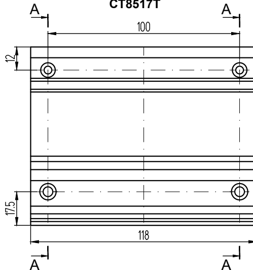
Обработка притвора створки СТ8517Т
