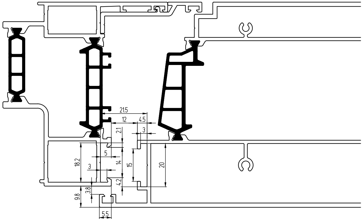
Размеры европаза 15/20 вентиляционных створок СТ85
