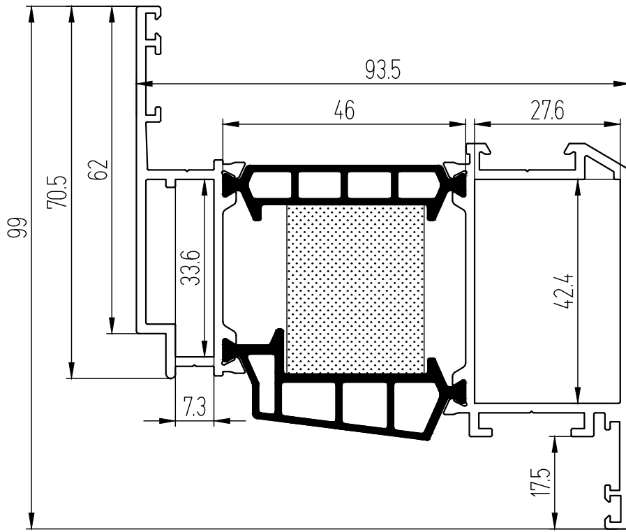
Штульп оконный (комбинированный) с термоизолирующим наполнителем
