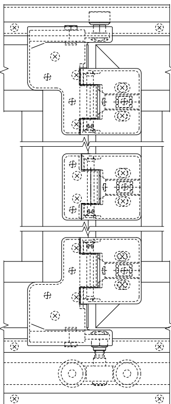
Узел С (нижняя тележка - несущая)
