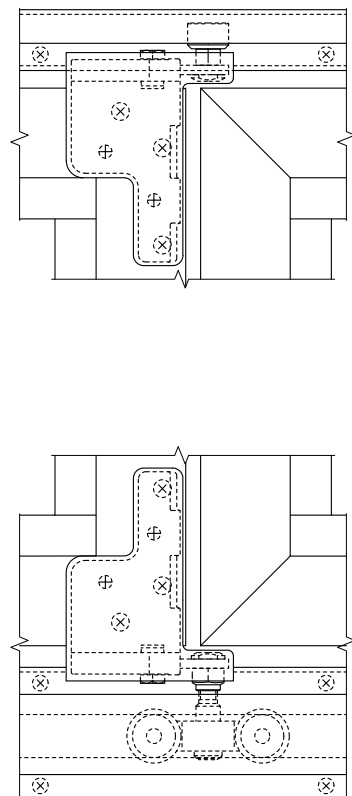
Узел D (нижняя тележка - несущая)
