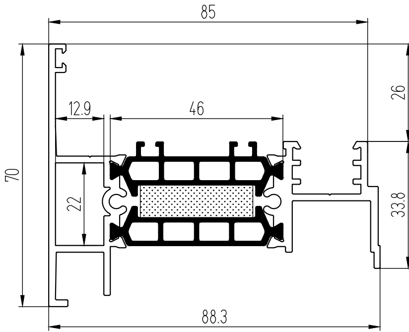
Штульп оконный (комбинированный) с термоизолирующим наполнителем
