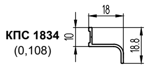
Отлив на петли
