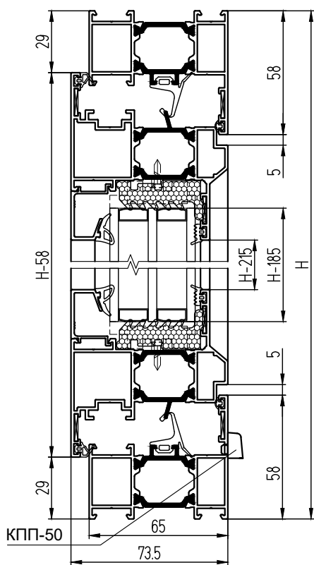
СТ65 Б-Б (1:2,5)
