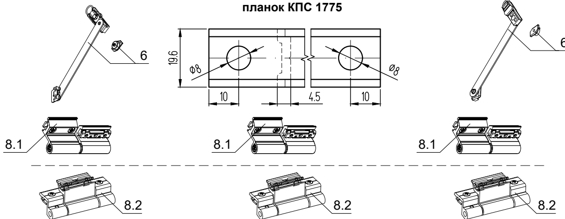
Обработка передвижных панок КПС 1775
