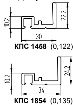
Держатели дверей
