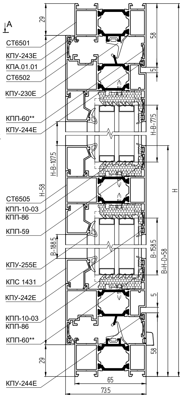
СТ65 А-А (1:2,5)
