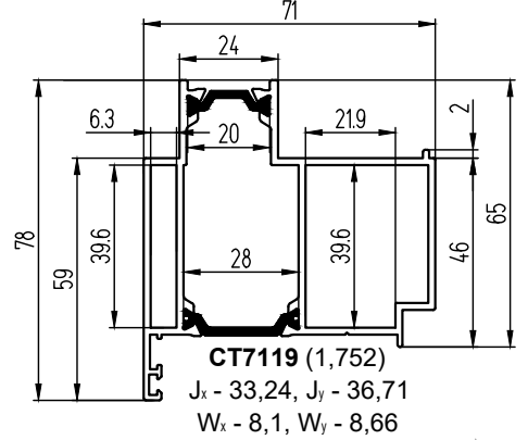
Рама в фасад
