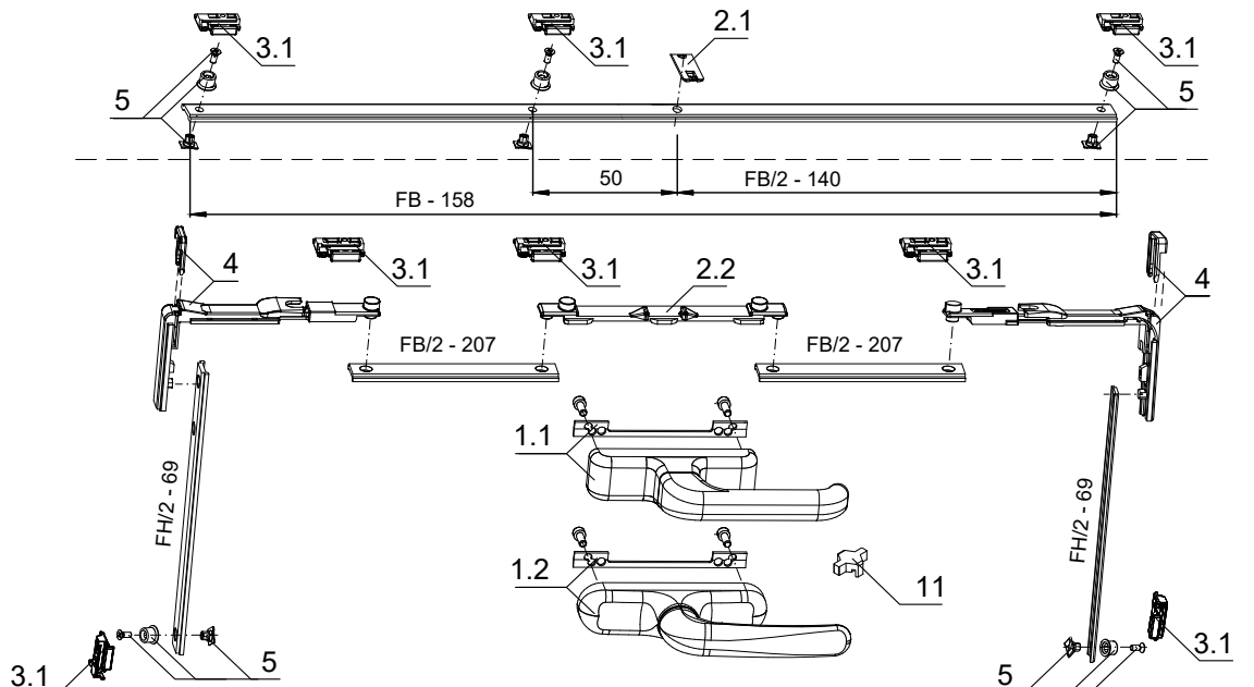
Обработка передвижных панок КПС 1775
