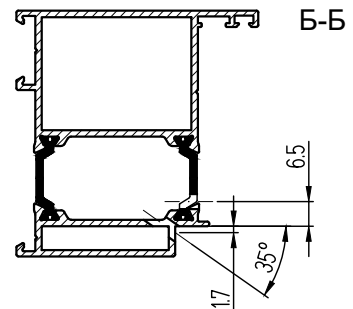
Обработка стойки рамы двери при установке петель Dr. Hahn „Rollenband AT“
