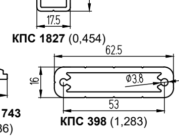
Держатель тяжелых стеклопакетов
