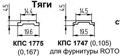
Закладные дверей со скрытыми петлями
