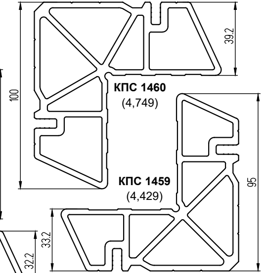
Стойчатые закладные
