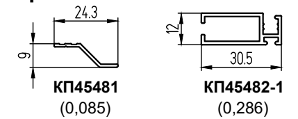
Профили противомоскитных сеток
