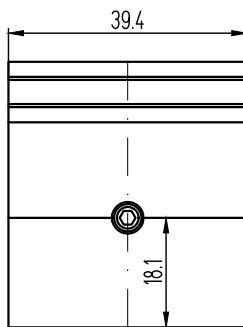
КПС 1424-39,4
