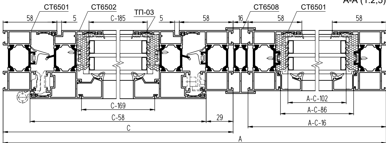
СТ65 А-А (1:2,5)
