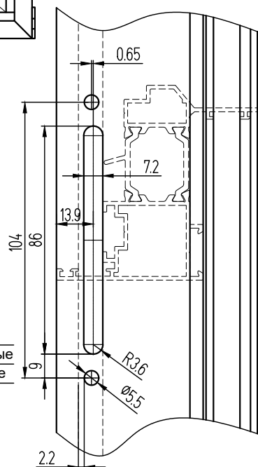
Обработка стойки створки СТ6504/СТ7104/СТ71104 под установку ручки
