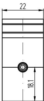
КПС 1424-22
