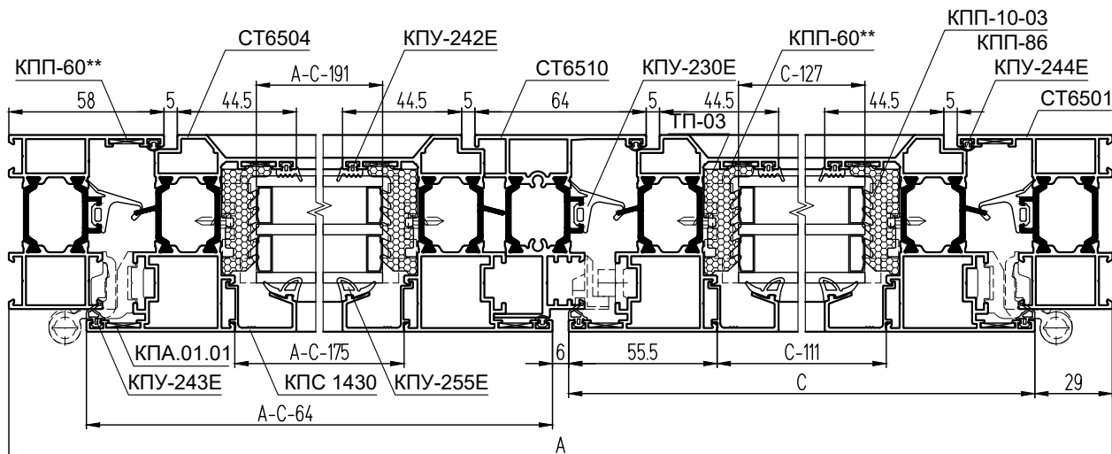
СТ65 А-А (1:2,5)
