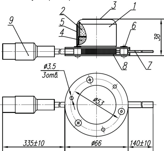
Рис.1. Генератор огнетушащего аэрозоля «Допинг 2.02»
