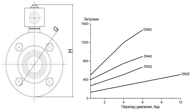
Диаграмма 1. Зависимость расхода от давления
