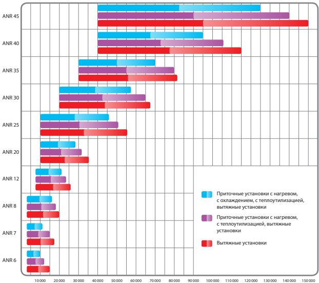
Воздухопроизводительность
