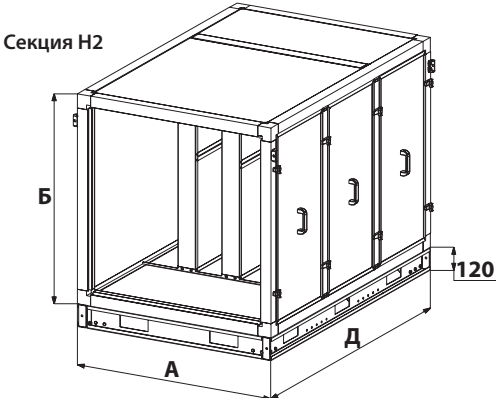
Н1 Н2 секция шумоглушения удлиненная секция шумоглушения
