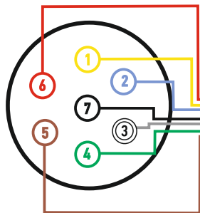
Розетка фаркопа
