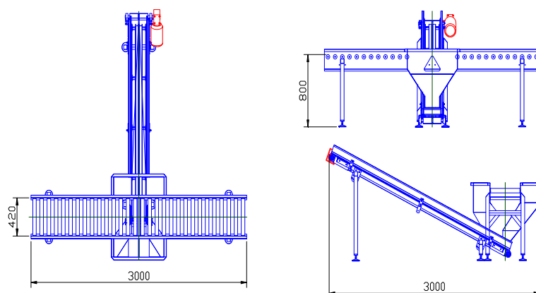
Размеры СТО-40
