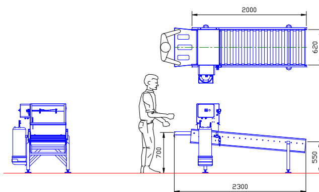
Размеры VU-15-T
